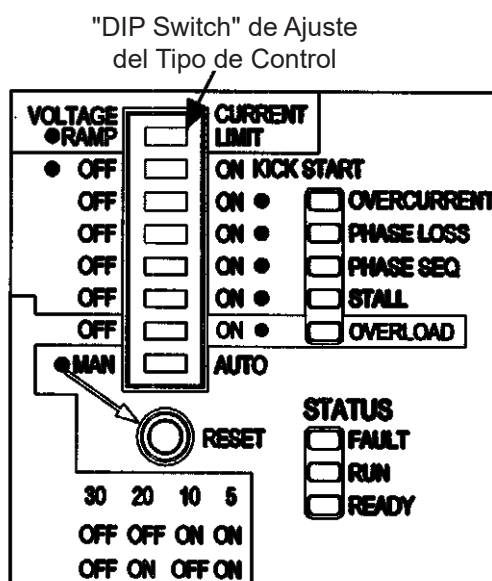
Figura 4.1 - Ajuste del tipo de control
