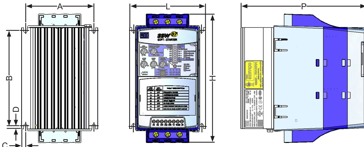
Figura 3.1 - Dimensional da SSW-07
