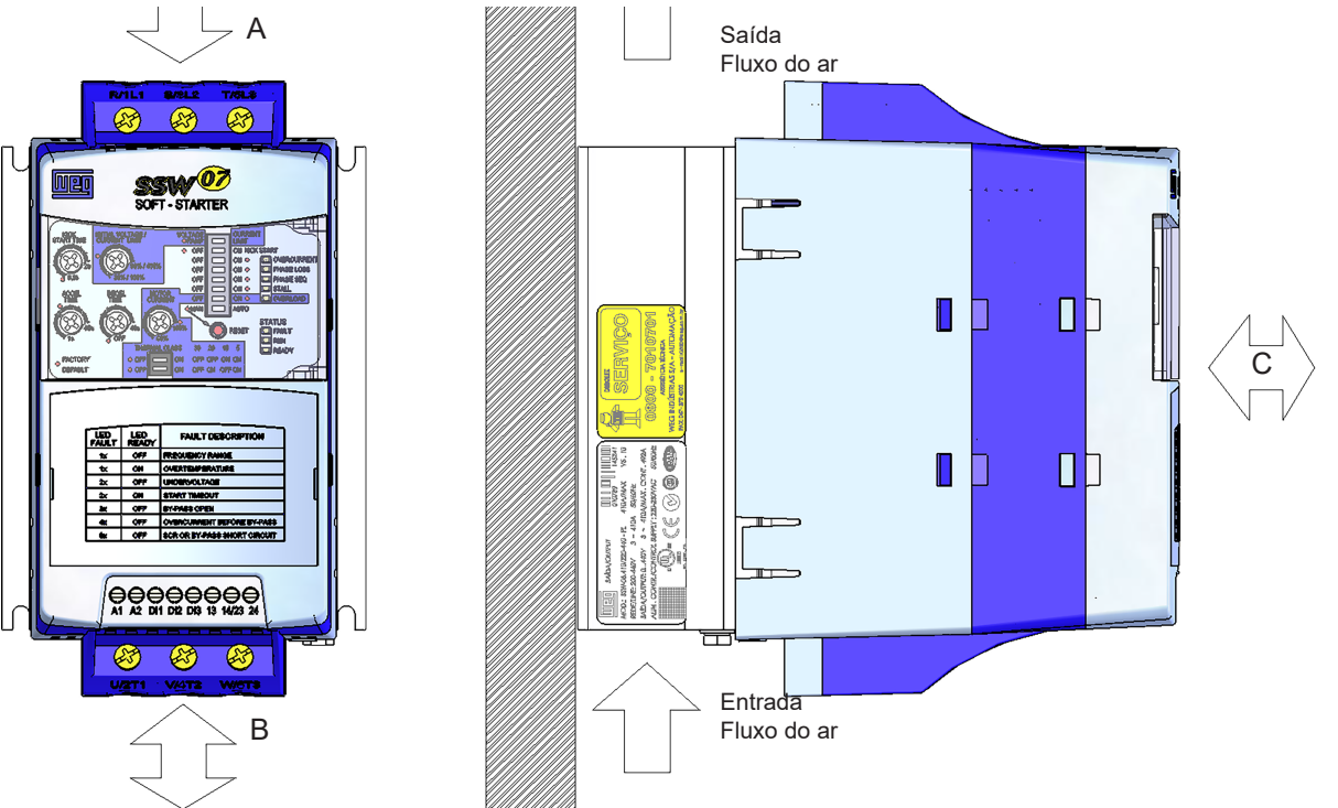
Figura 3.2 - Espaços livres para ventilação
