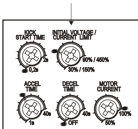
Figura 4.4 - Ajuste do limite de corrente
