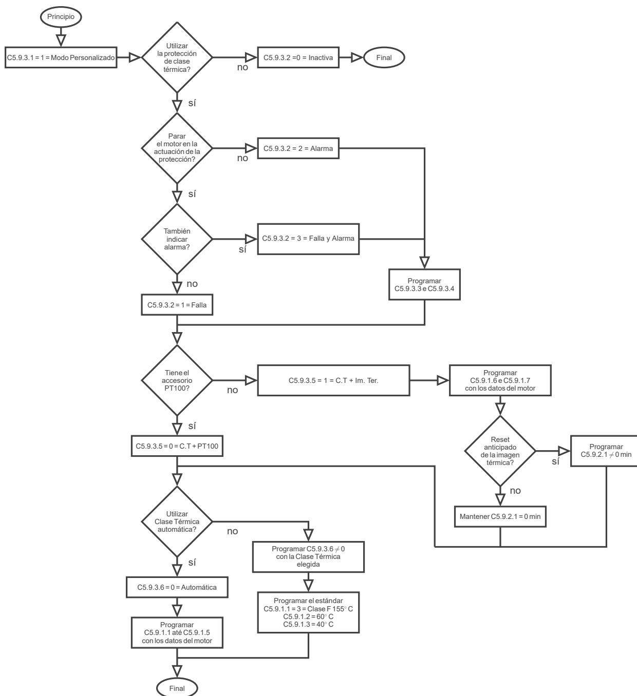
Figura 11.28: Secuencia de programación de la Protección de Clase Térmica modo personalizado.
