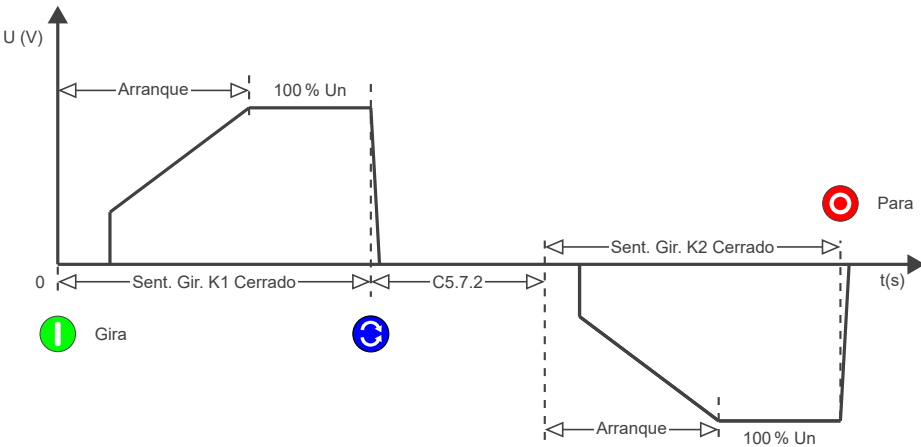
Figura 11.30: Cambio del Sentido de Giro vía Contactor.
