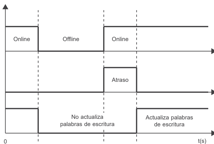
Figura 11.38: Atraso en la actualización de las palabras de I/O
