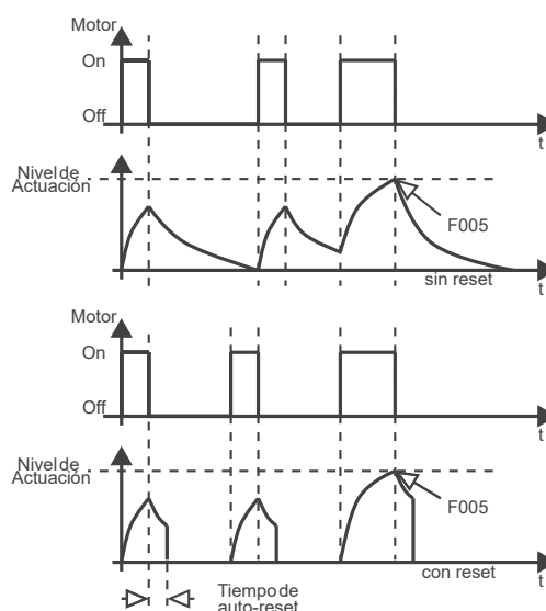
Figura 11.26: Reset de la imagen térmica del motor.
