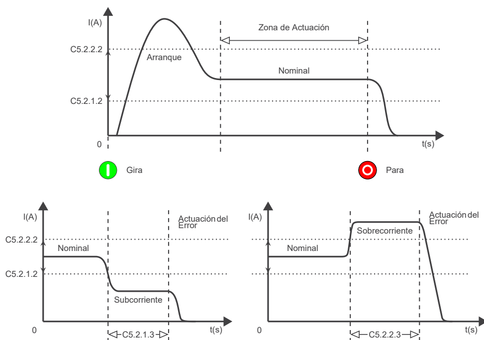
Figura 11.16: Niveles de actuación para sobre y subcorriente.
