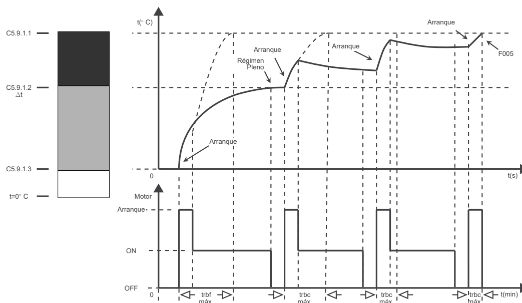
Figura 11.23: Calentamiento del motor.
