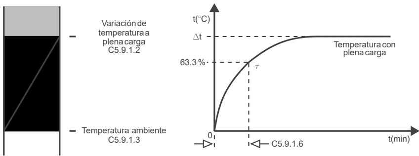
Figura 11.24: Constante de calentamiento del motor para corriente nominal.
