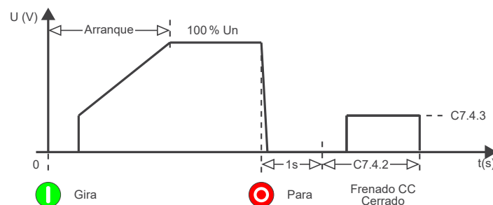
Figura 11.36: Frenado CC.
