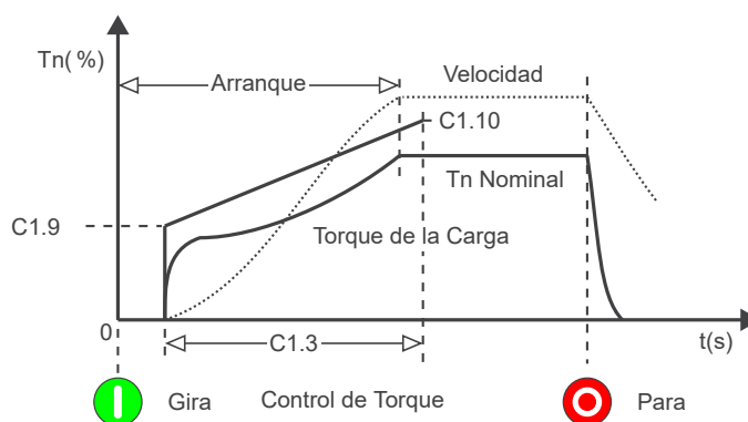
Figura 13.15: Arranque con Control de Torque Lineal, 2 puntos, Carga Cuadrática.
