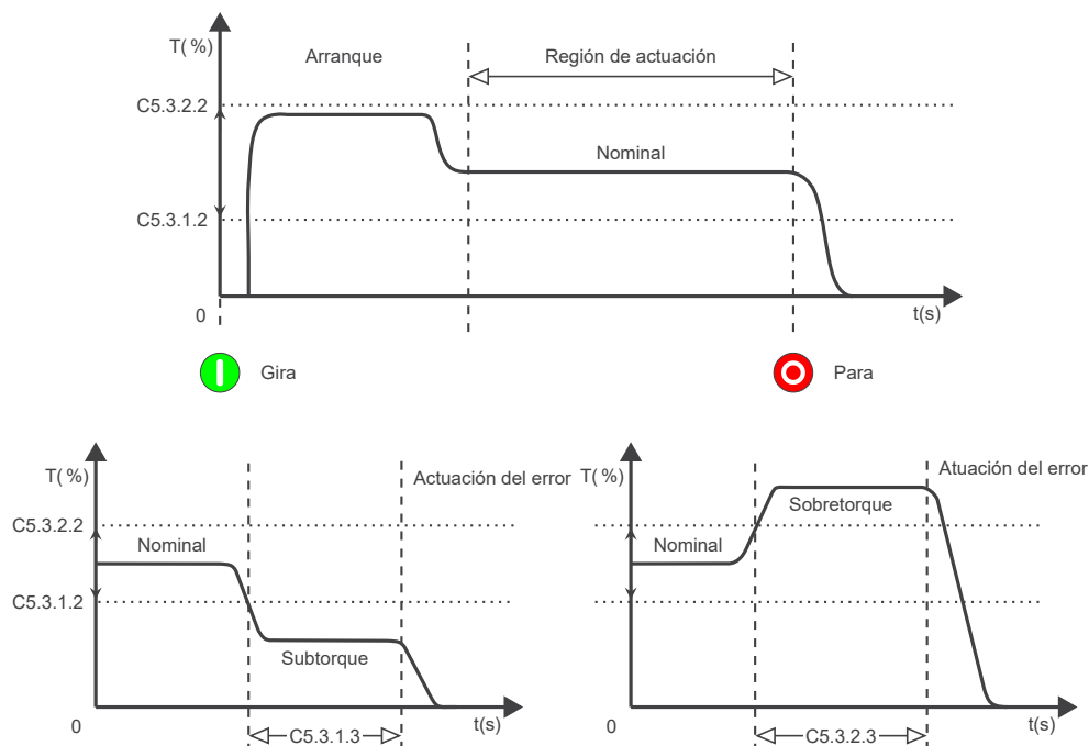
Figura 11.17: Niveles de Actuación para Sobre y Subtorque.
