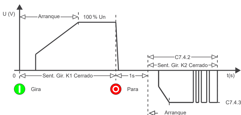
Figura 11.34: Frenado por reversión.
