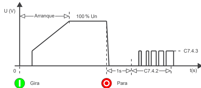
Figura 11.35: Frenado óptimo.
