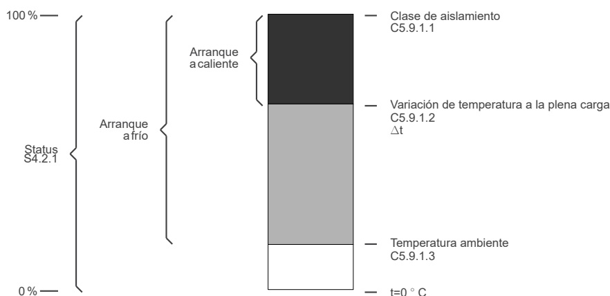
Figura 11.22: Rangos de temperatura del motor dentro de la clase de aislamiento.
