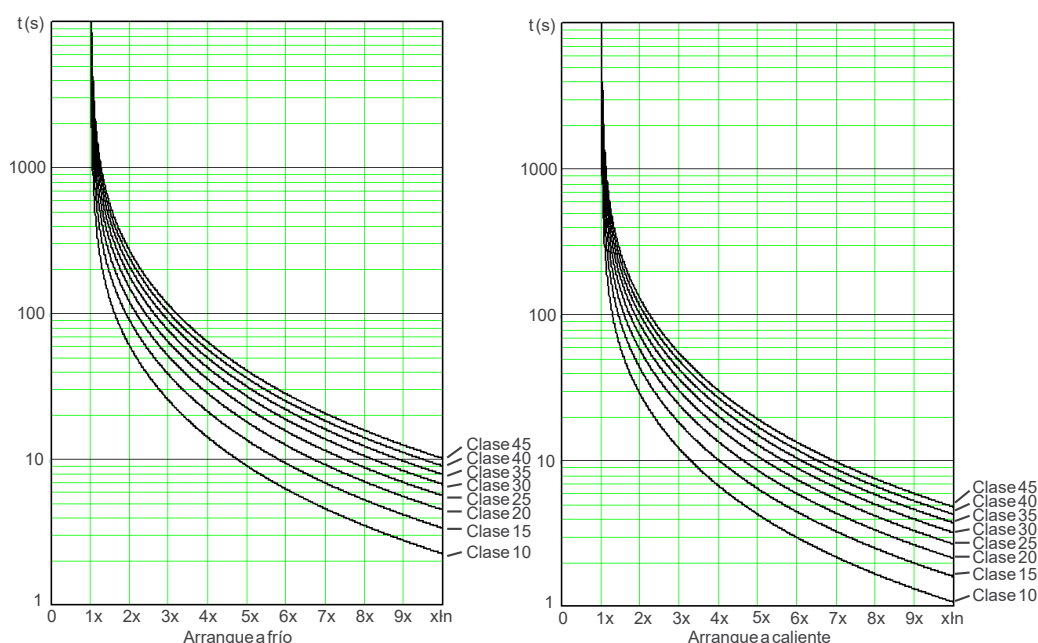
Figura 11.29: Clases Térmicas de Protección del Motor estándar.
