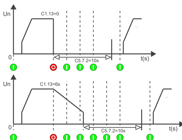
Figura 11.18: Accionamiento vía HMI.
