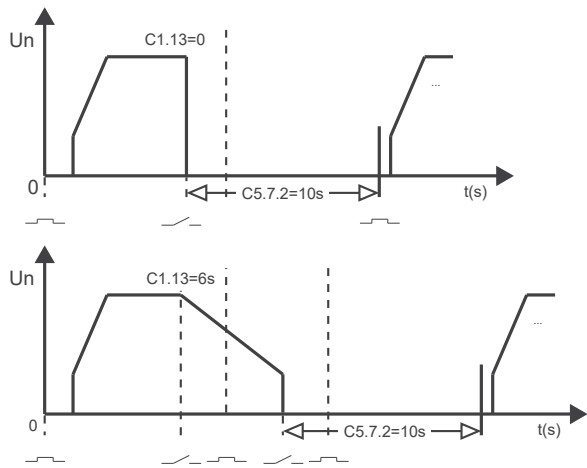
Figura 11.20: Accionamiento vía entrada digital (DI1).
