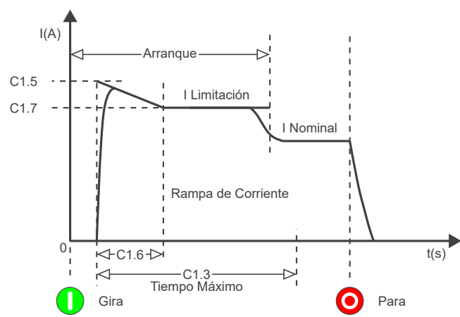
Figura 11.6: Límite de Corriente por Rampa de Corriente en el Arranque más Alto.
