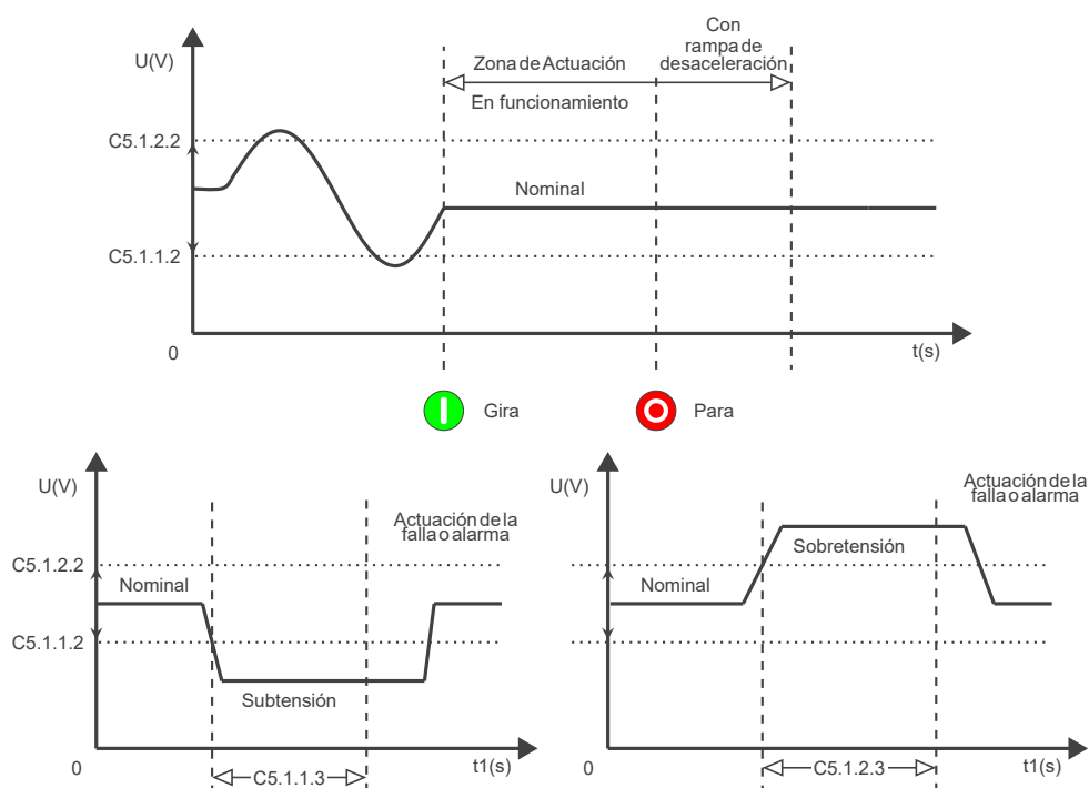
Figura 11.14: Niveles de actuación de la sobre y subtenión.
