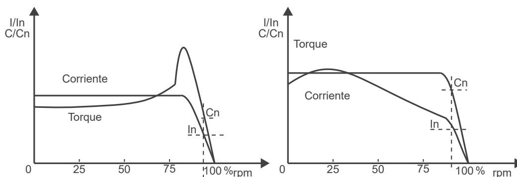
Figura 13.2: Curvas características de torque y de corriente en un arranque con Limitación de corriente y por Control de Torque.
