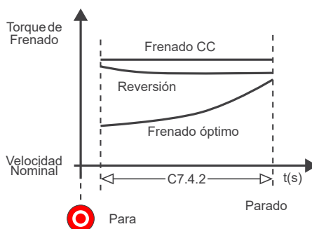
Figura 11.33: Torque de frenado.
