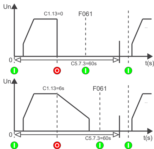
Figura 11.21: Tiempo entre arranques.
