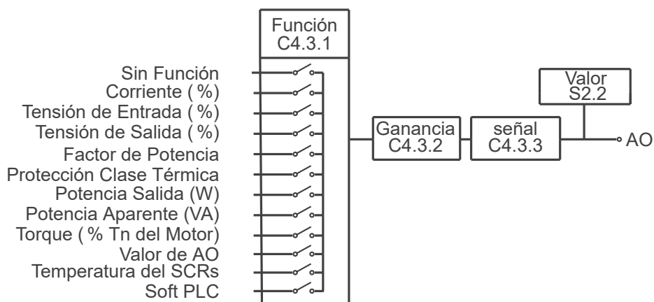
Figura 11.12: Diagrama de Bloques de las Salidas Analógicas.
