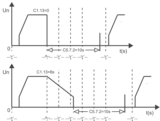
Figura 11.19: Accionamiento vía entradas digitales a tres cables (DI1 y DI2).
