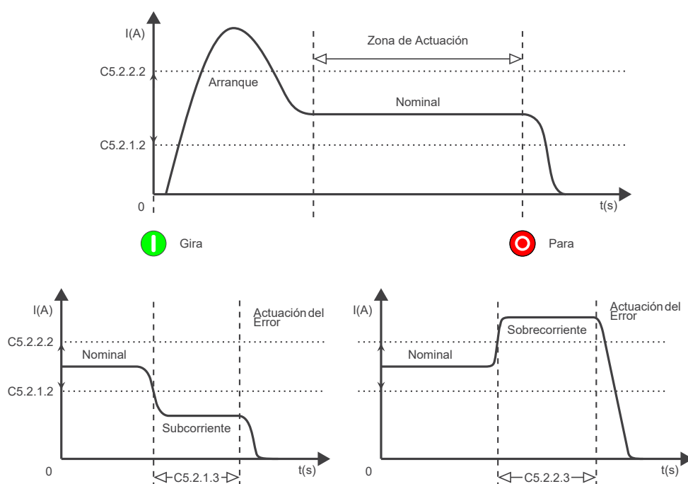
Figura 11.15: Niveles de actuación para sobre y subcorriente.
