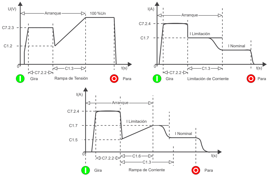
Figura 11.32: Niveles de Actuación del Pulso de Torque en el Arranque.
