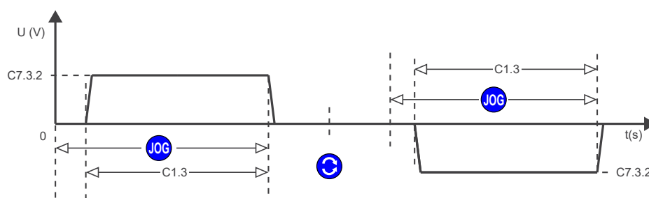
Figura 11.31: Cambio de Sentido de Giro Sólo para JOG.
