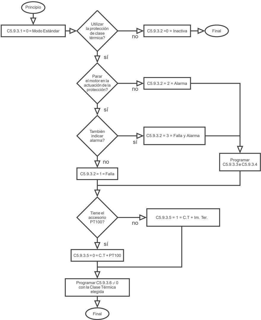
Figura 11.27: Secuencia de programación de la Protección de Clase Térmica modo estándar.
