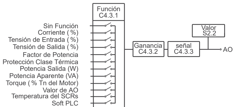
Figura 11.13: Diagrama de Bloques de las Salidas Analógicas.
