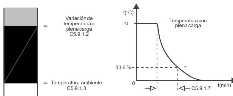
Figura 11.25: Constante de enfriamiento del motor desenergizado.
