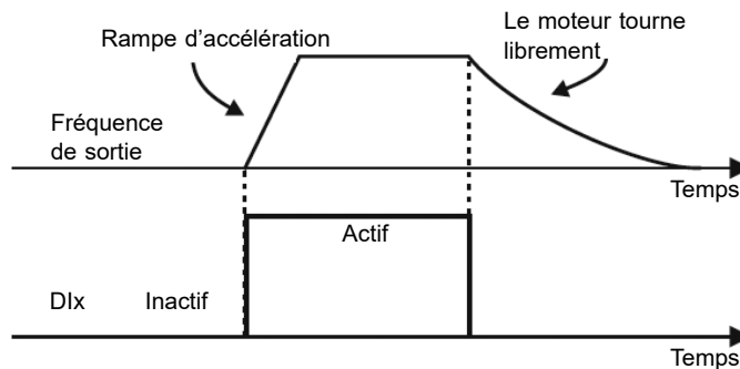
Figure 9.7 : Exemple de la fonction Activation générale
