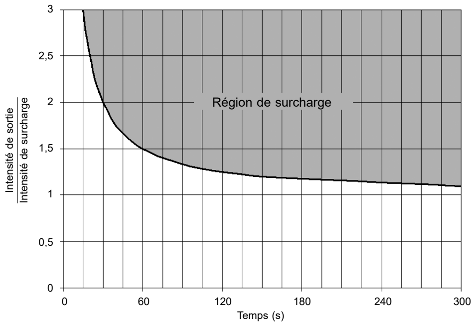
Figure 10.2 : Activation de la surcharge du moteur
