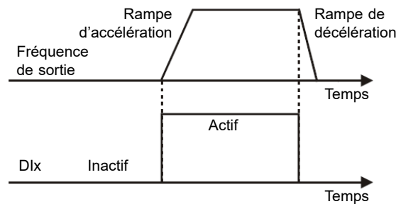
Figure 9.6 : Exemple de la fonction Marche/arrêt
