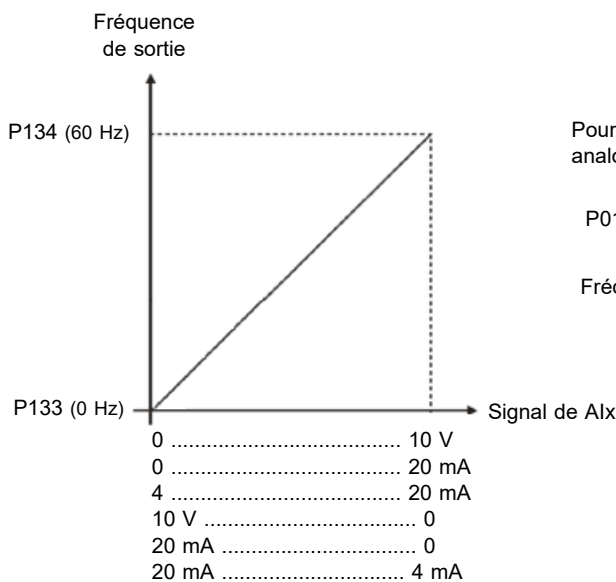
Figure 15.2 : Résultat pour l'application 1
