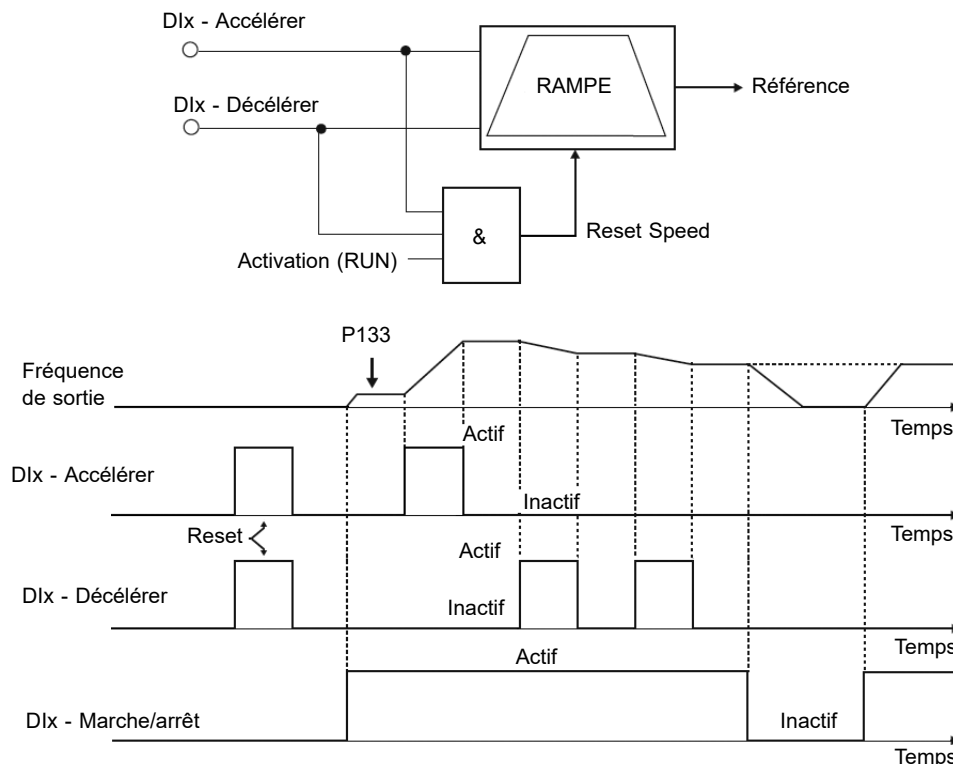
Figure 9.13 : Exemple de la fonction Potentiomètre électronique (E.P.)
