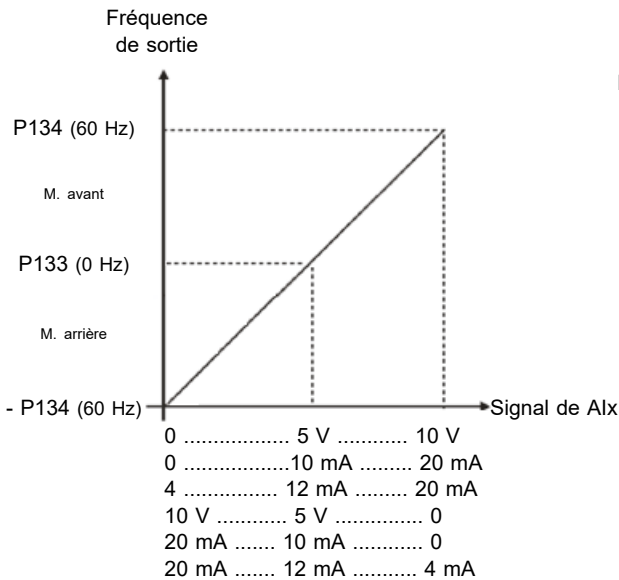
Figure 15.4 : Résultat pour l'application 3
