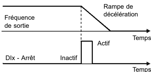
Figure 9.17 : Exemple de la fonction Arrêt
