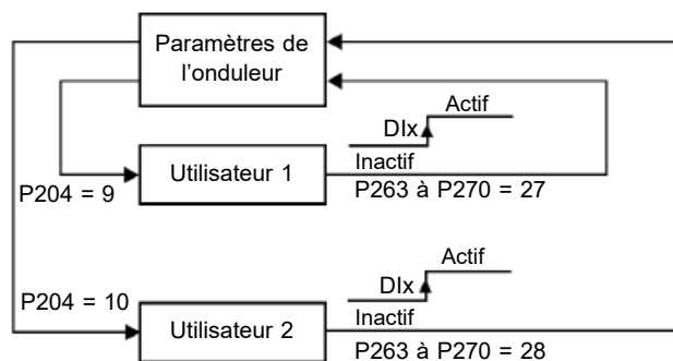
Figure 9.15 : Schéma fonctionnel des charges de fonctions utilisateur 1 et utilisateur 2
