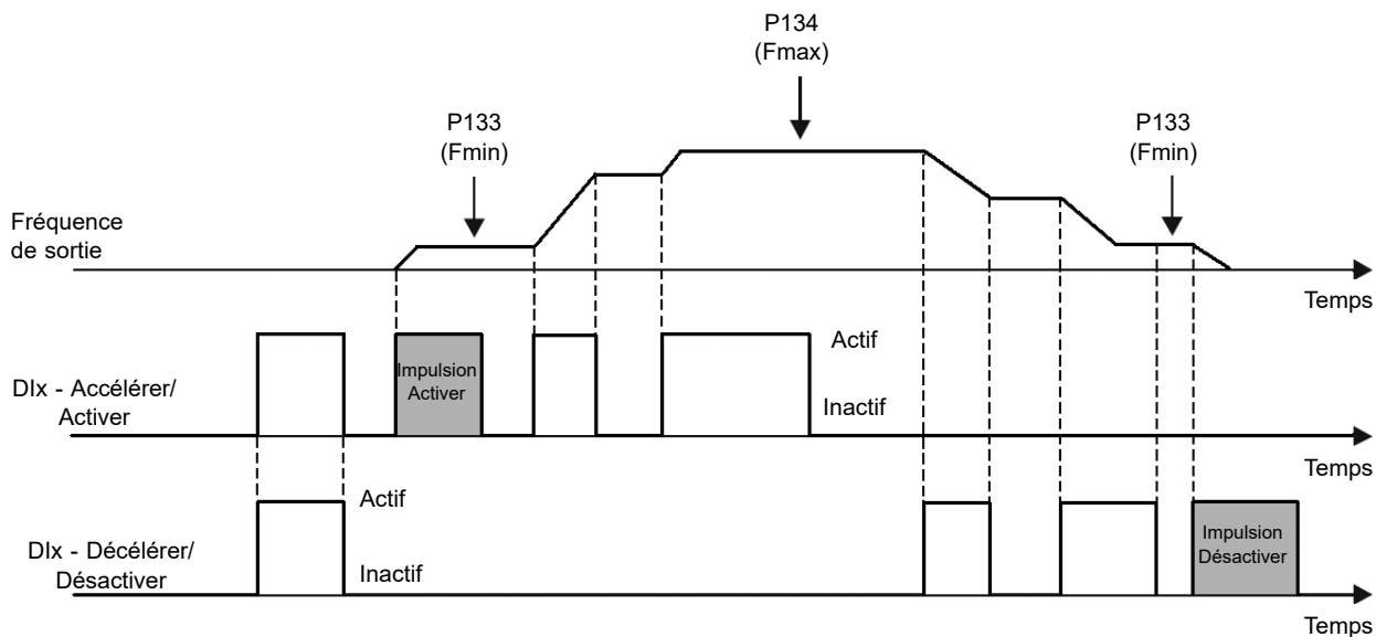
Figure 9.16 : Exemple de Activer l'accélération / Désactiver décélération
