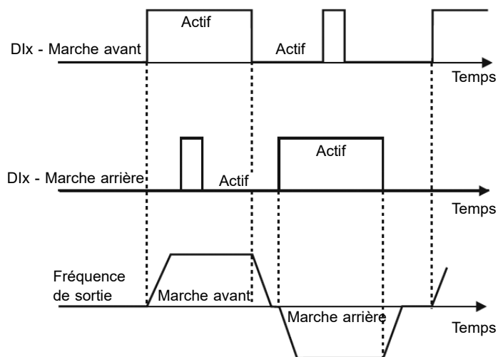
Figure 9.9 : Exemple de la commande Marche avant/arrière
