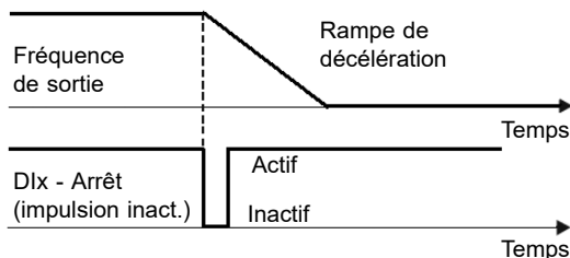
Figure 9.18 : Exemple de fonction d'arrêt avec impulsion inactive
