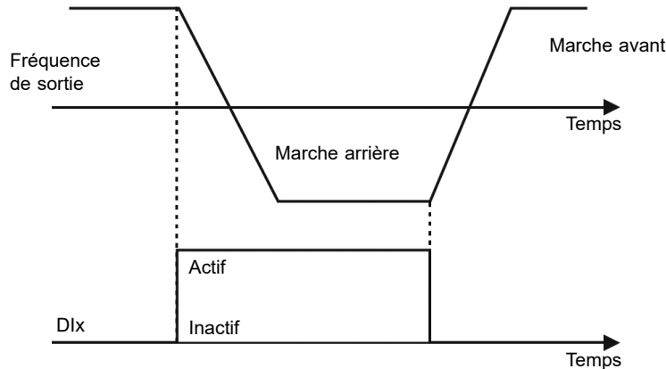
Figure 9.11 : Exemple de la fonction Sens de rotation
