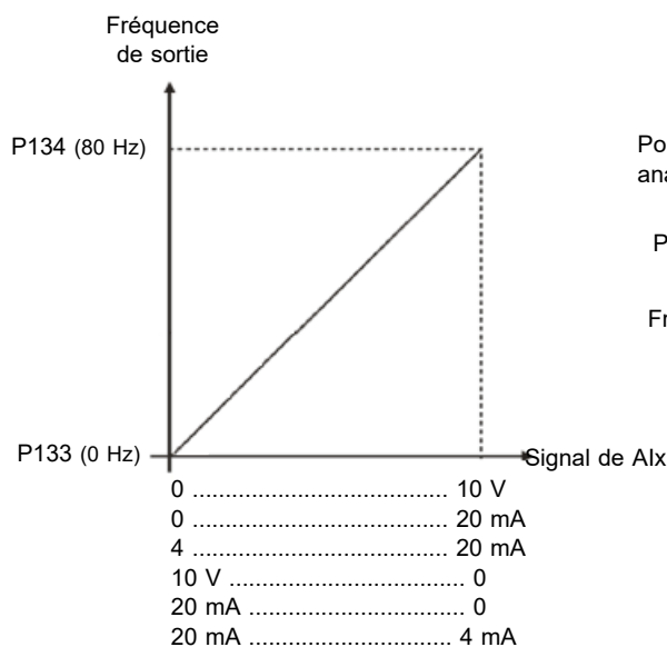
Figure 15.3 : Résultat pour l'application 2
