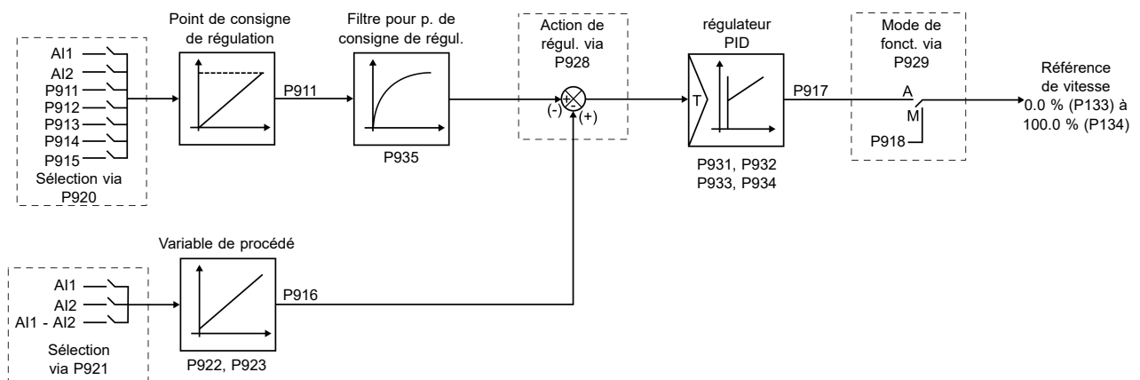
Figure 14.1 : Schéma de principe du régulateur PID
