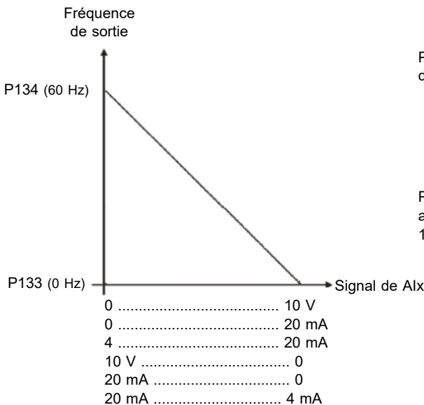
Figure 15.6 : Résultat pour l'application 5
