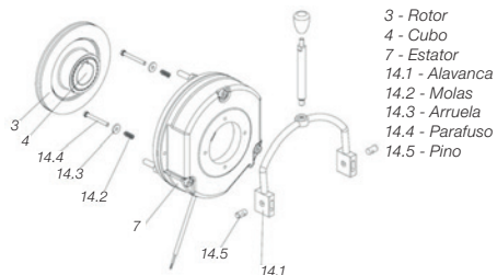
Figura 10 - Componentes que compõem a alavanca de destravamento
