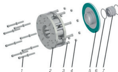
Figura 4 - Componentes do freio eletromagnético - tamanho 25 e 31 (800 a 2.400 Nm)
