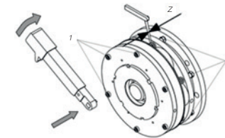
Figura 7 - Verificação do entrefreio nos freios de tamanhos 25 e 31
