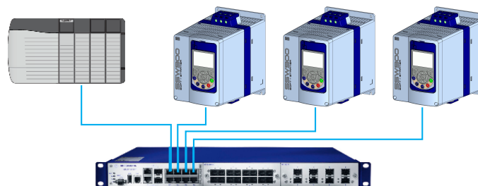
Figura 3.1: Topologia estrela
