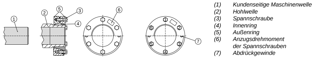
Abbildung 5: Hohlwelle mit Schrumpfscheibe
