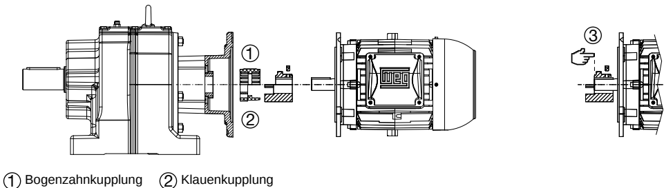
Abbildung 12: Montage eines IEC-Motors an einen Kupplungsadapter
