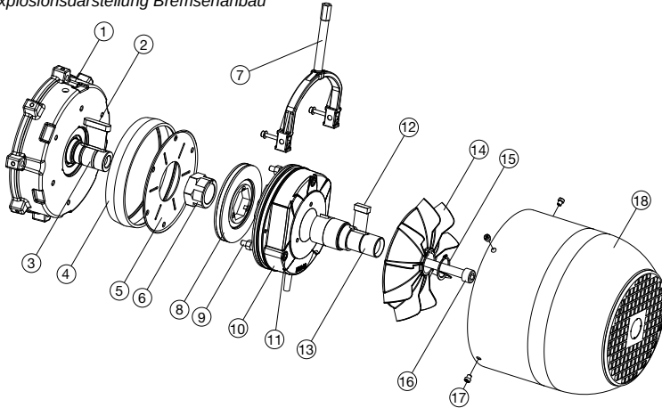
Abbildung 18: Explosionsdarstellung Bremsenanbau
