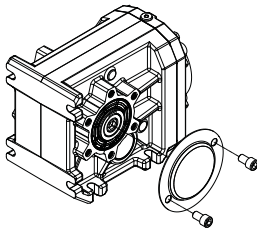
Abbildung 6: Getriebe mit Hohlwellen-Abdeckkappe
