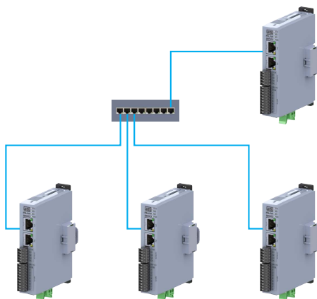
Figura 3.2: Topología en estrella
