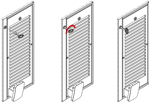
Figura 4.11: Instrucciones para apertura de las puerta frontal
