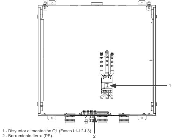
Figura 5.2: Conexiones de los cables de alimentación - Fases (L1-L2-L3) y puesta a tierra (PE)
