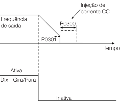
Figura 14.7: Atuação da Frenagem CC
