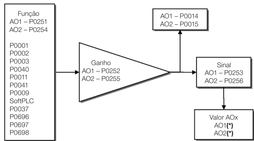
(*) Bornes de controle disponíveis no módulo Plug-in. Figura 15.3: Diagrama de blocos das saídas analógicas – AOx
