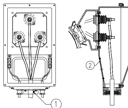
Figura 4.6: Caixa de ligação
