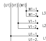
Figura 4.9: Conexões paralelas
