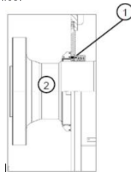
Figura 8.1: Medição entreferro
