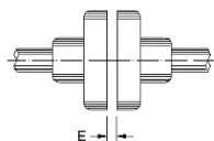
Figura 4.16: Folga axial do acoplamento (E)
