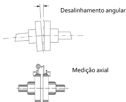
Figura 4.14: Alinhamento angular
