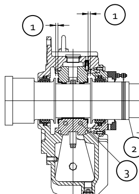
Figura 4.18: Mancal de deslizamento
