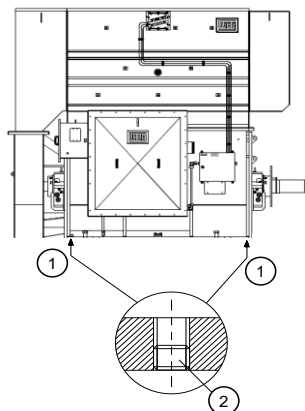
Figura 3.2: Dreno do motor
