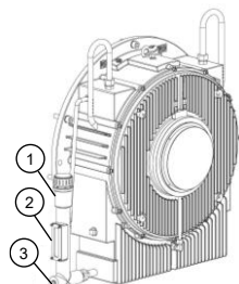
Figura 7.3: Mancal de rolamento a óleo
