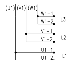
Figura 4.8: Conexões paralelas
