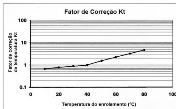
Figura 4.3: Fator de correção da resistência de isolamento em função da temperatura
