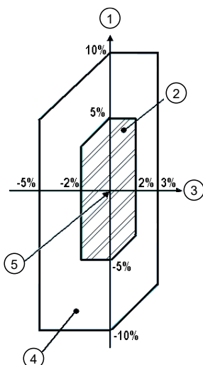
Figura 2.1: Limites das variações de tensão e frequência
