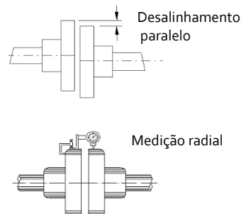
Figura 4.13: Alinhamento paralelo
