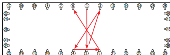
Figura 4.4: Informação de aperto
