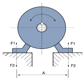
Figura 4.10: Esforços nas fundações
