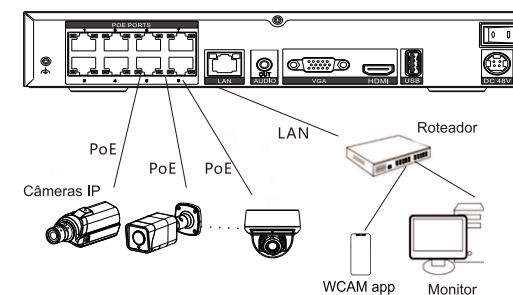
Figura 6-1 Gravador NVR
