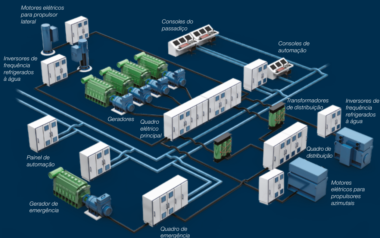
Diagrama de automação para navios diesel-elétricos
