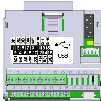
Figura 2.3: Módulo plug-in con conexión USB
