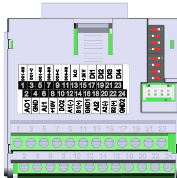
Figura 2.2: Módulo plug-in con RS485 adicional
