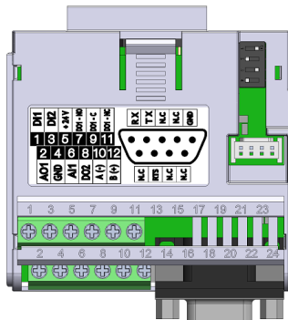
Figura 2.4: Módulo plug-in con conexión RS232
