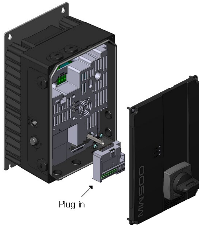
Figura 2.1: Ejemplo de accesorio de interfaz para MW500
