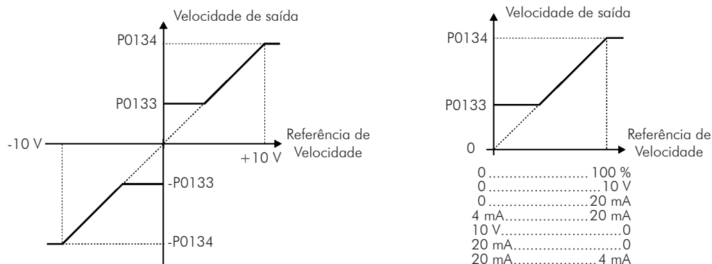
Figura 12.3 - Limites de velocidade considerando "Zona Morta" ativa (P0230=1)
