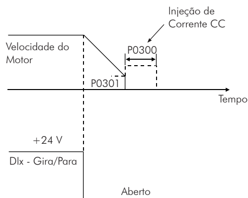
Figura 12.11 (b) - Atuação da frenagem CC no bloqueio por rampa (via desabilita rampa) (cont.)
