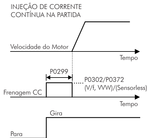
Figura 12.10 - Atuação de frenagem CC na partida
