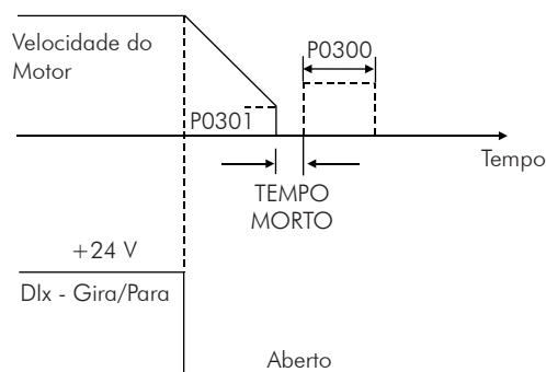
Figura 12.11 (a) - Atuação da frenagem CC no bloqueio por rampa (via desabilita rampa)
