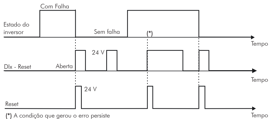
Figura 13.6 (h) a (j) - Detalhes sobre funcionamento das funções das entradas digitais (cont.)
