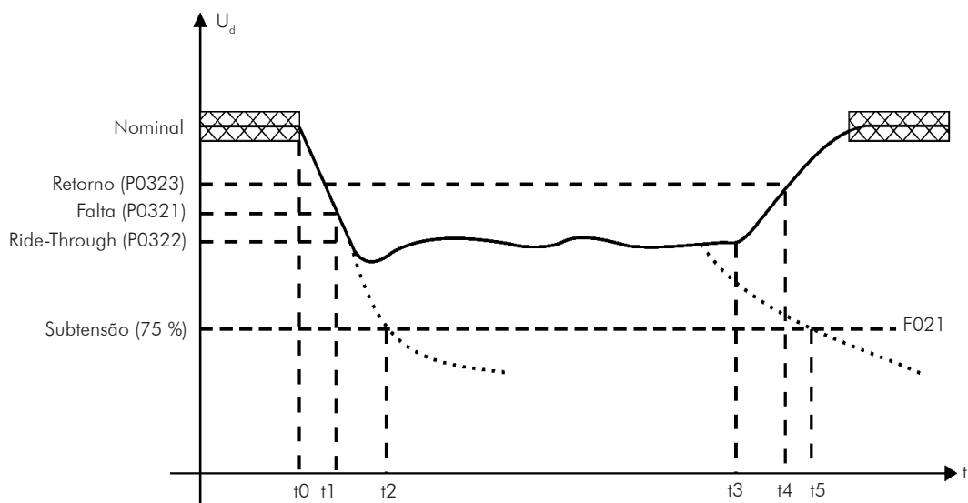
Figura 12.8 - Atuação da função Ride-Through em modo vetorial
