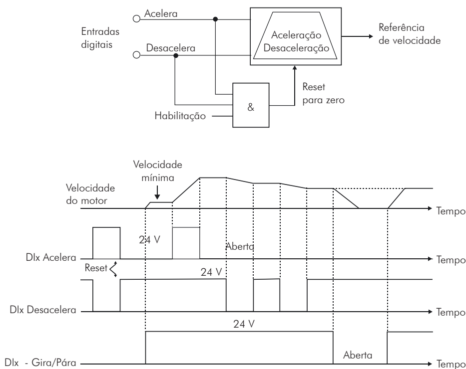
Figura 13.6 (k) a (m) - Detalhes sobre funcionamento das funções das Entradas digitais (cont.)
