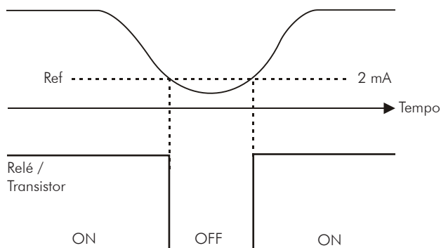
Figura 13.7 (e) a (k) - Detalhes do funcionamento das funções das saídas digitais e a relé (cont.)
