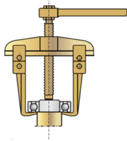
Рисунок 7.3. Съемник подшипников качения
