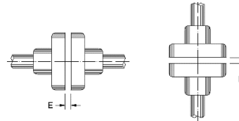
Рисунок 4.12. Осевой зазор муфты (E)
