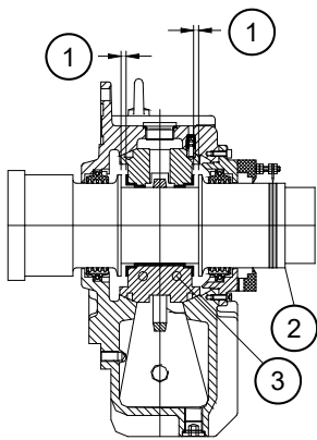
Рисунок 4.14. Подшипник скольжения
