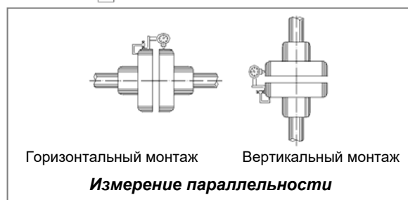
Рисунок 4.9. Регулировка соосности
