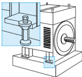
Рисунок 4.8. Анкерные болты
