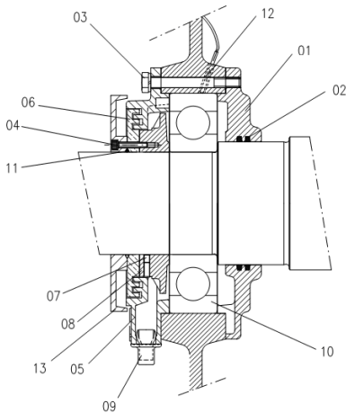
Рисунок 7.6. Детали подшипника качения с консистентной смазкой
