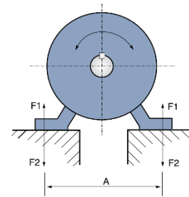
Рисунок 4.6. Нагрузка на основание
