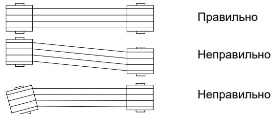
Рисунок 4.13. Ременный привод
