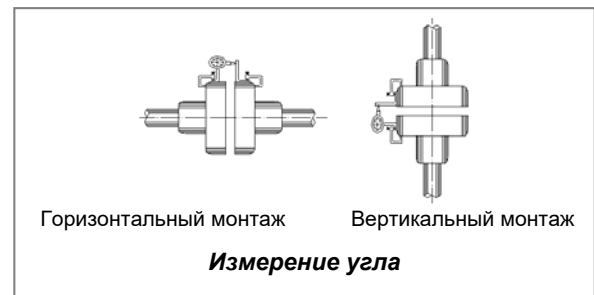
Рисунок 4.10. Угловое выравнивание
