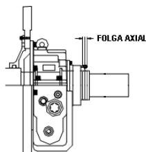
Figura 4.17: Marcação do centro magnético
