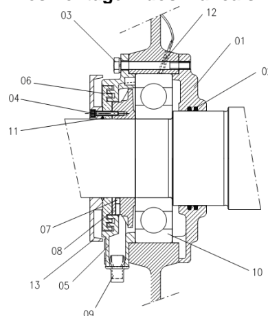
Figura 7.6: Partes do mancal de rolamento a graxa
