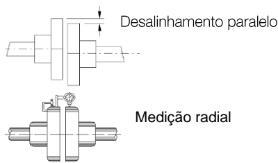
Figura 4.11: Alinhamento paralelo
