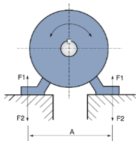
Figura 4.8: Esforços nas fundações
