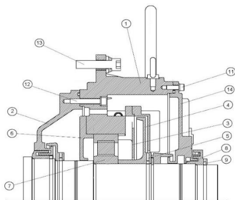
Figura 7.9: Partes do mancal de rolamento a óleo
