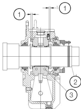
Figura 4.16: Mancal de deslizamento
