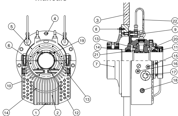
Figura 7.11: Partes do mancal de deslizamento
