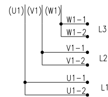
Figura 4.6: Conexões paralelas
