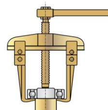
Figura 7.10: Dispositivo para sacar o rolamento
