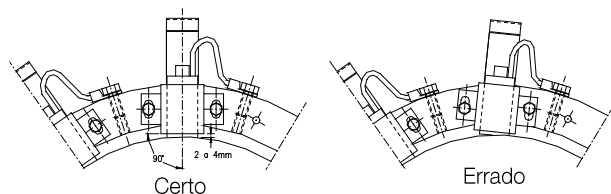
Figura 7.3: Montagem do porta escovas
