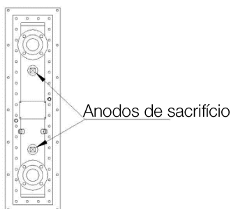
Figura 4.5: Radiador com anodos de sacrifício
