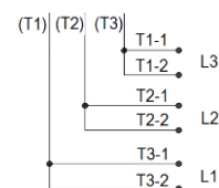
Figura 4.7: Conexões paralelas
