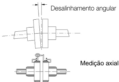
Figura 4.12: Alinhamento angular
