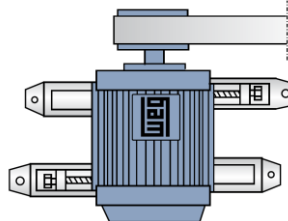
Figura 4.9: Base deslizante
