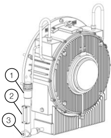
Figura 7.8: Mancal de rolamento a óleo
