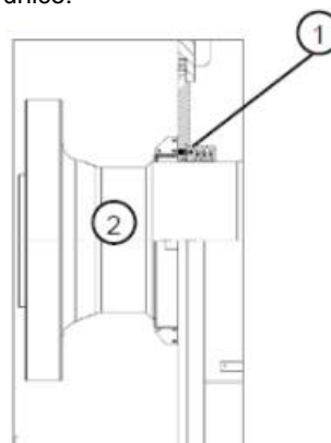
Figura 8.1: Medição entreferro
