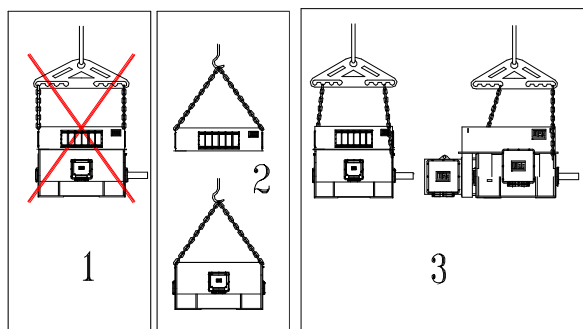
Figura 3.1: Manuseio dos motores
