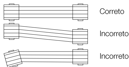
Figura 4.15: Acoplamento por polias e correias
