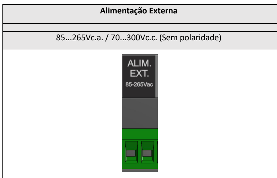
Figura 4 - Alimentação Externa
