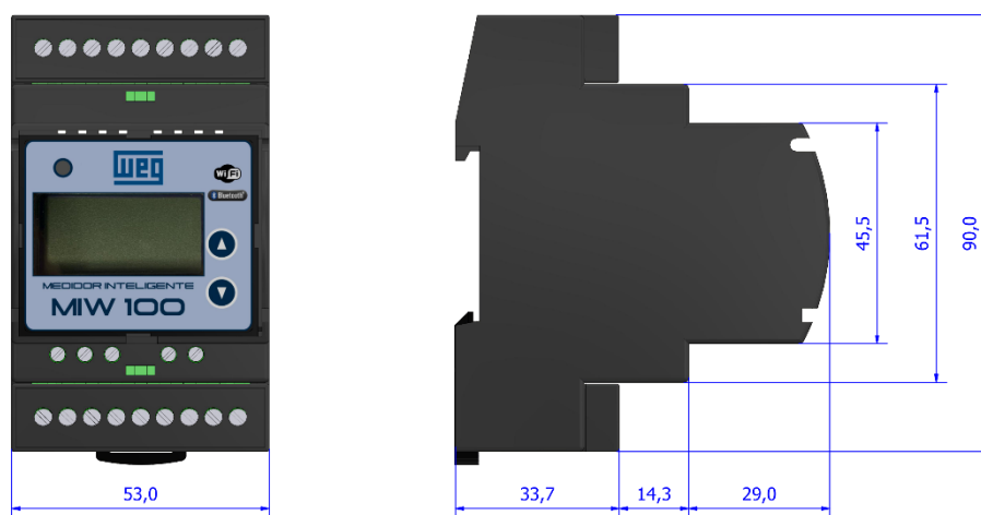
Figura 2 - Dimensionais
