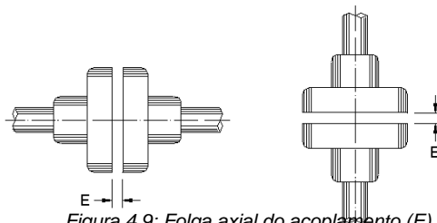
Figura 4.9: Folga axial do acoplamento (E)
