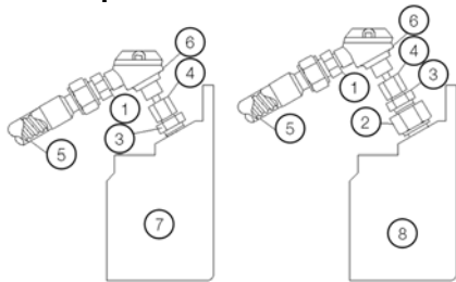
Figura 7.5: Pt100 nos mancais
