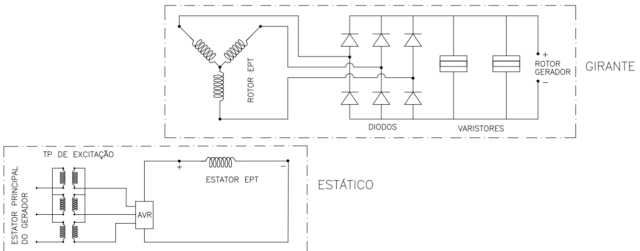
Figura 5.2: Circuitos elétricos internos do gerador sem PMG
