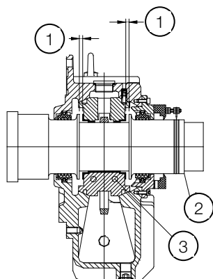
Figura 4.10: Mancais de deslizamento
