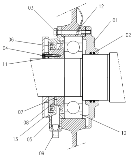
Figura 7.1: Partes do mancal de rolamento a graxa
