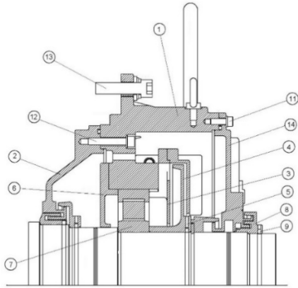
Figura 7.4: Partes do mancal de rolamento a óleo
