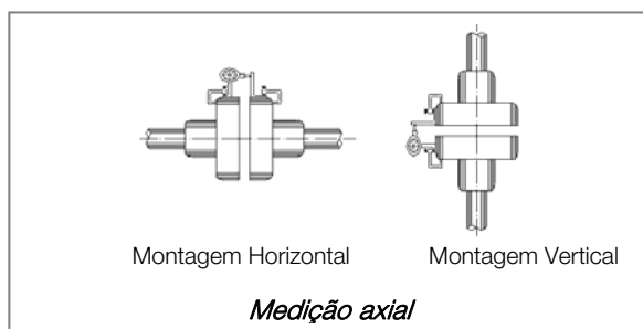
Figura 4.7: Alinhamento angular
