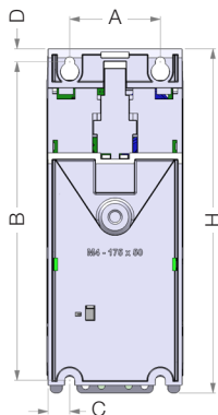
Wymiary podstawy montażowej
