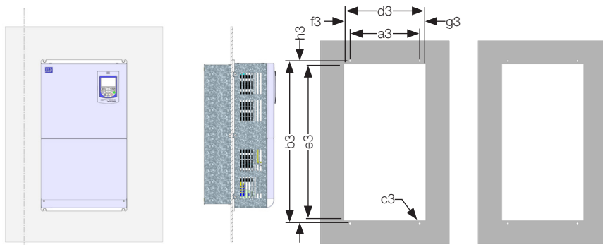
(c) Montaż kołnierzy - falownik standardowy (tylko rozmiary ramy F, G)
