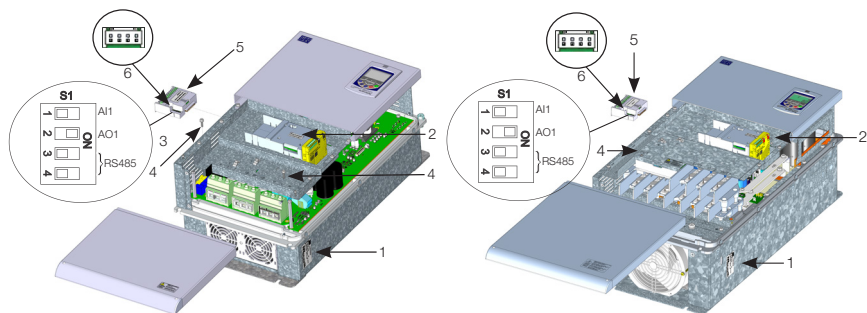
Rozmiar ramy F
