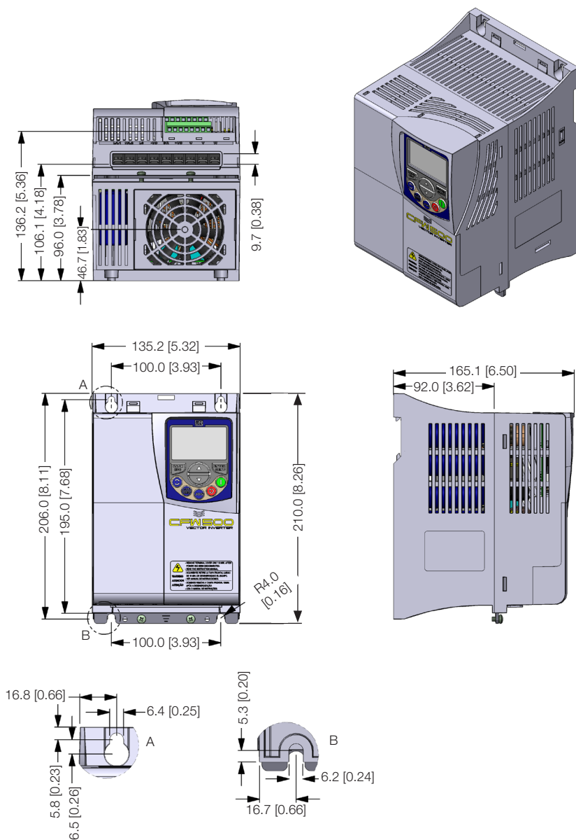
Rysunek B.7: Wymiary przetwornicy w mm [in] – rozmiar obudowy C
