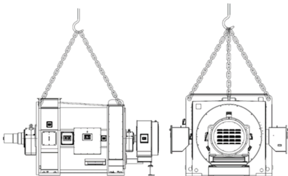
Figura 3.1: Manuseio - geradores IM1001/1005
