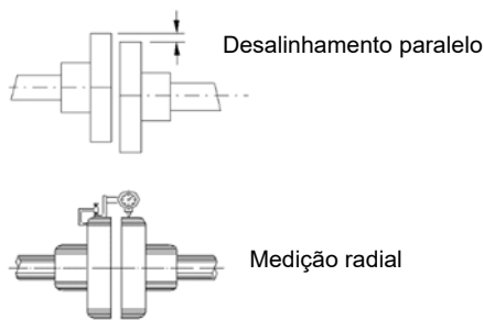
Figura 4.5: Alinhamento paralelo
