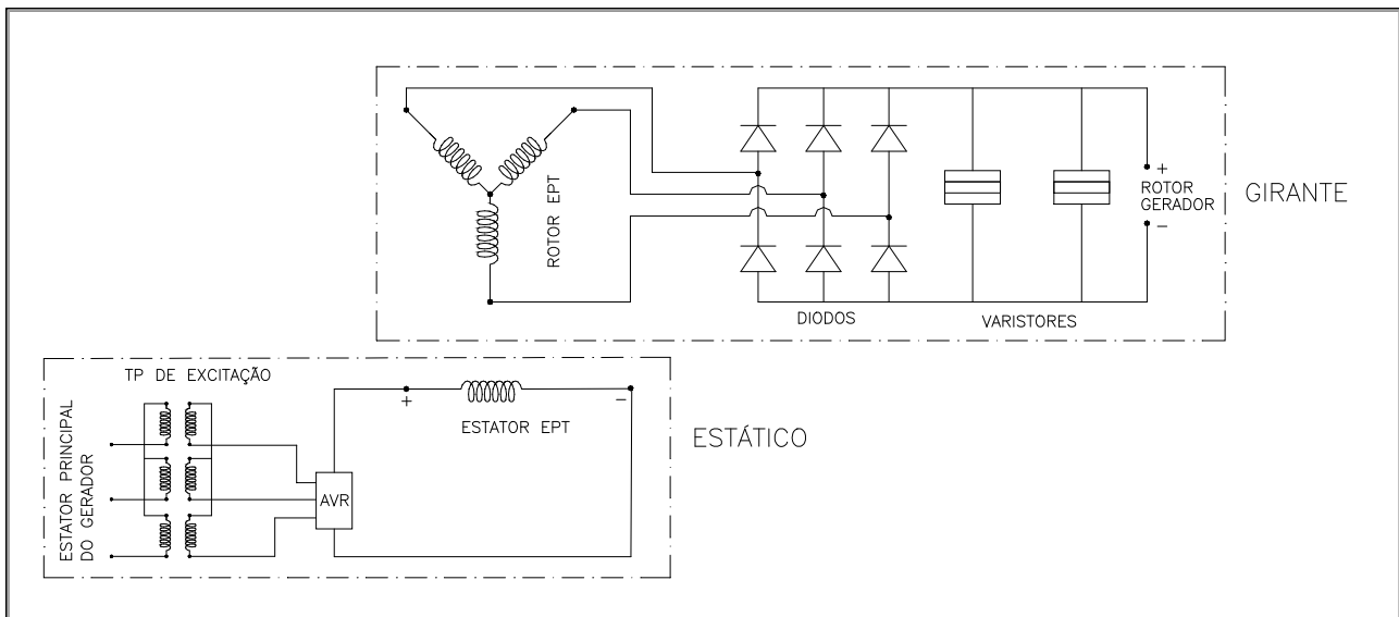
Figura 5.2: Circuitos elétricos internos do gerador sem PMG
