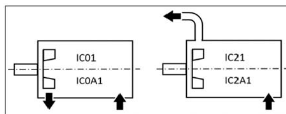
Figura 4.4: Refrigeração
