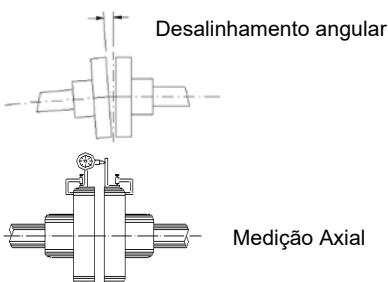
Figura 4.6: Alinhamento angular
