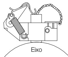
Figura 7.1: Escova para aterramento do eixo
