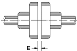
Figura 4.8: Folga axial do acoplamento (E)
