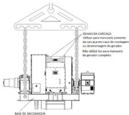
Figura 3.2: Manuseio - geradores IM7311/7315.
