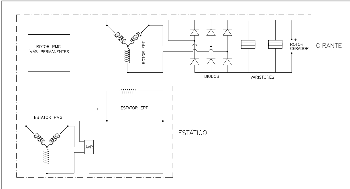
Figura 5.1: Circuitos elétricos internos do gerador com excitatriz auxiliar (PMG)
