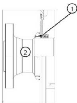
Figura 8.1: Medição entreferro
