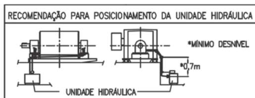
Figura 4.11: Unidade hidráulica
