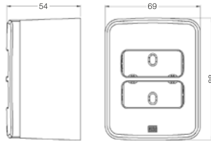
Caixa e placa de sobrepor 2 posições
