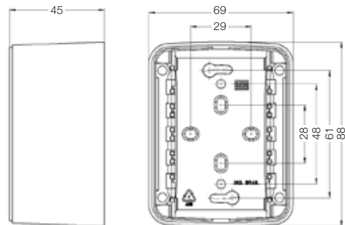
Caixa de sobrepor
