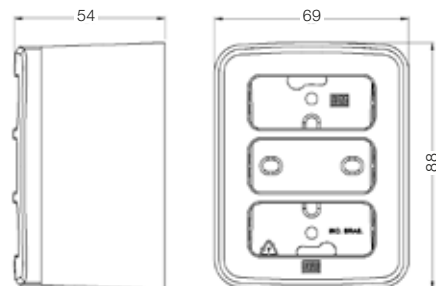
Caixa e placa de sobrepor 3 posições
