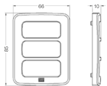
Placa sobrepor 3 posições
