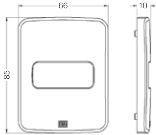
Placa sobrepor 1 posição
