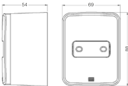
Caixa e placa de sobrepor 1 posição
