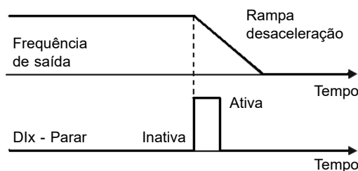
Figura 9.16: Exemplo da função Parar
