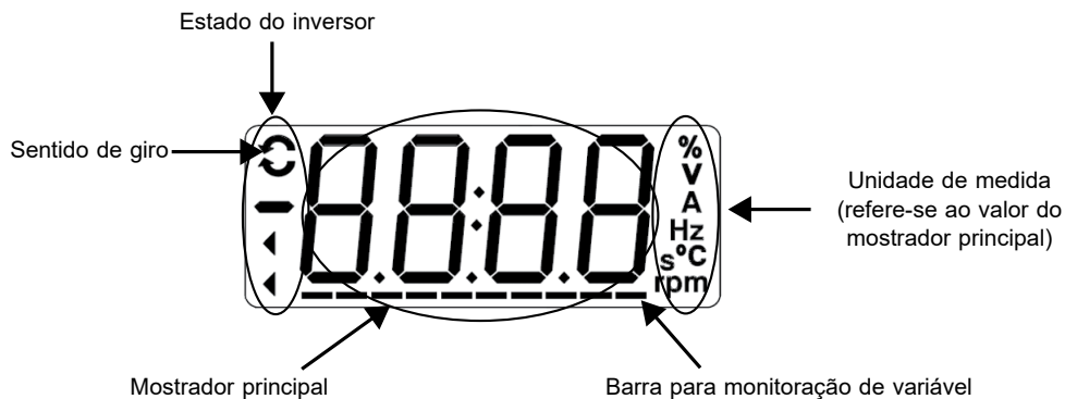
Figura 4.2: Áreas do display
