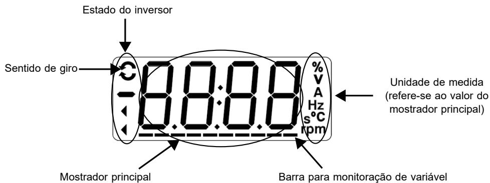
Figura 5.1: Tela na inicialização e campos do display
