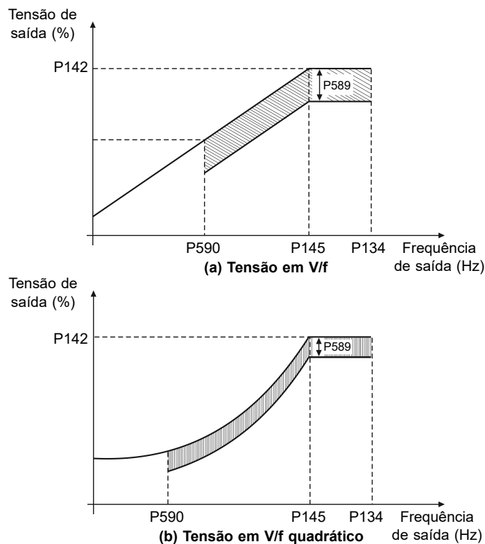
Figura 8.19: (a) e (b) Exemplo de comportamento da tensão em V/f e V/f quadrático
