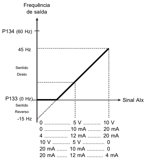
Figura 15.5: Resultado para aplicação 4
