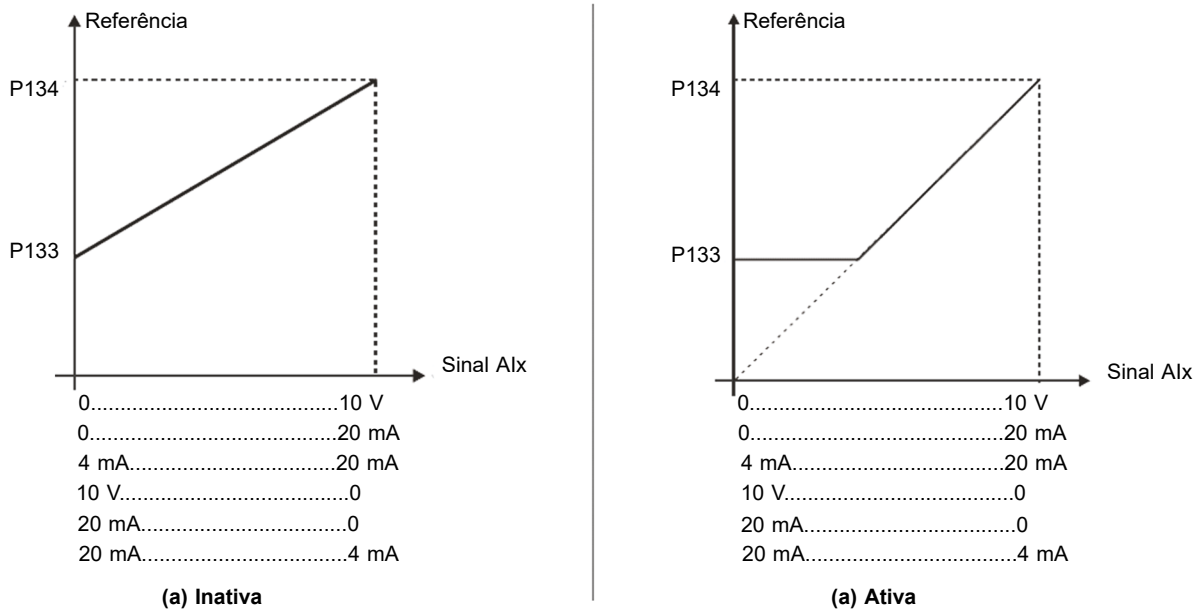
Figura 9.2: (a) e (b) Atuação da entrada analógica com zona morta
