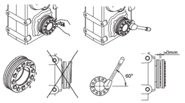
Figura 6 - Apriete del disco de contracción.
