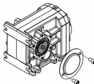
Figura 9 - Tapa de protección para el eje hueco.
