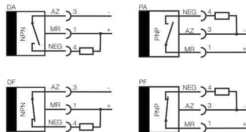
Figura 1: Diagrama eléctrico
