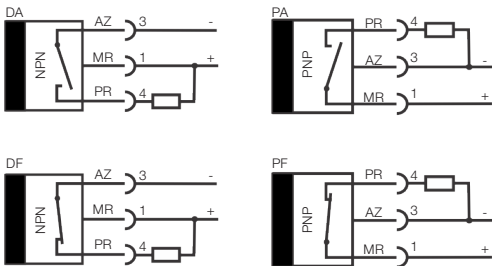
Figura 1: Diagrama elétrico
