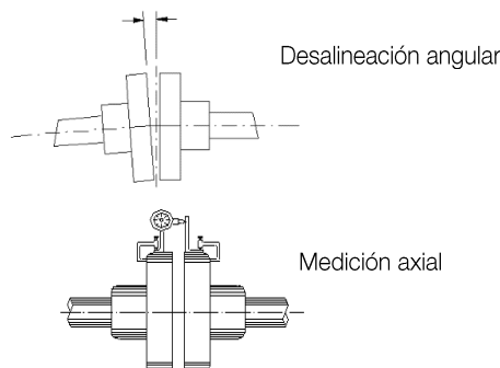
Figura 4.6: Alineación angular
