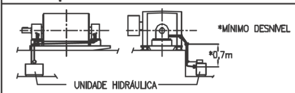
Figura 4.11: Unidad hidráulica
