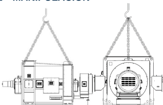
Figura 3.1: Manipulación - generadores IM1001/1005
