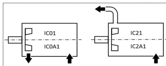
Figura 4.4: Refrigeración
