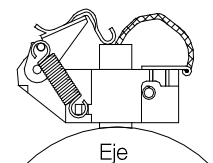
Figura 7.1: Escobilla para puesta a tierra del eje
