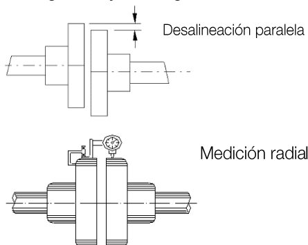
Figura 4.5: Alineación paralela
