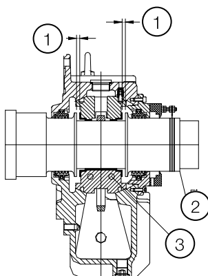
Figura 4.9: Cojinete de deslizamiento
