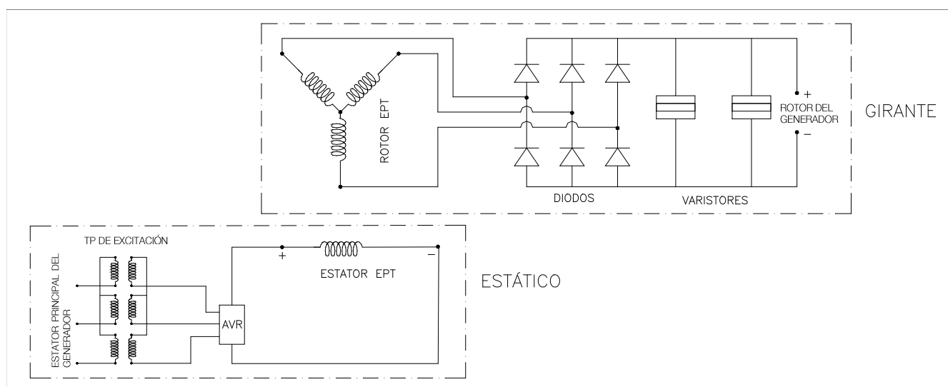
Figura 5.2: Circuitos eléctricos internos del generador sin PMG
