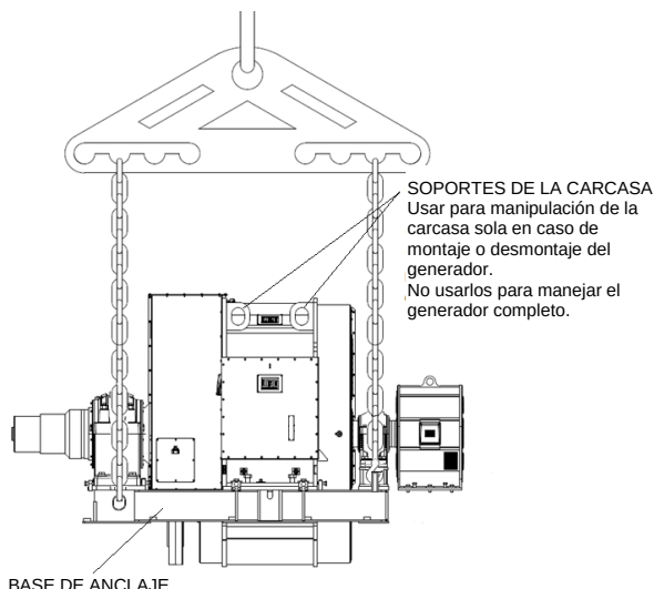
Figura 3.2: Manipulación - generadores IM7311/7315.
