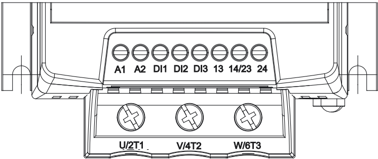
Figura 3.9: Bornes de controle da SSW-08
