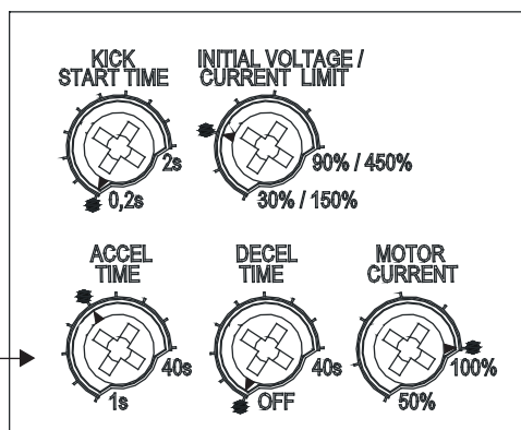
Figura 4.5: Ajuste do tempo da rampa de aceleração
