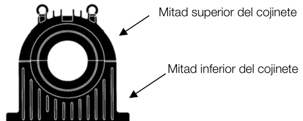
Figura 4.8: Cojinete de pedestal
