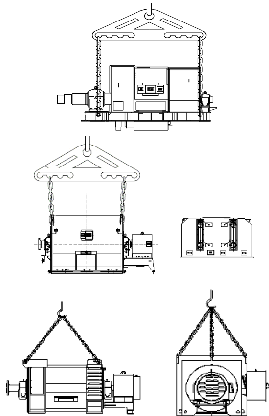
Figura 3.1: Manipulación de los generadores
