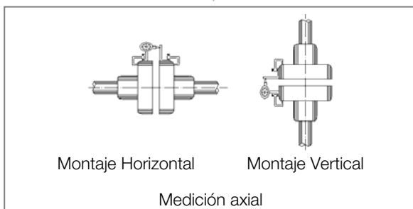
Figura 4.7: Alineación angular
