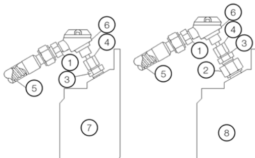
Figura 7.5: Pt100 en los cojinetes
