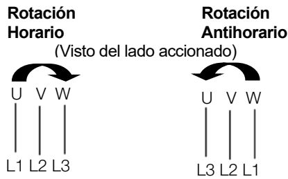
Figura 6.1: Secuencia de fases (IEC60034-8)
