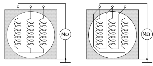
Figura 4.1: Conexión del megóhmetro
