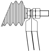
Figura 4.5: Conexión de cables paralelos
