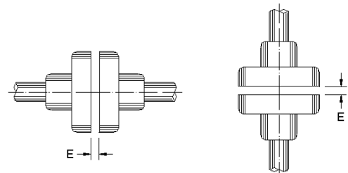
Figura 4.9: Holgura axial del acoplamiento (E)
