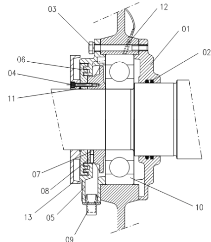
Figura 7.1: Partes del cojinete de rodamiento a grasa
