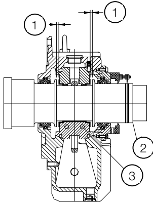
Figura 4.10: Cojinete de deslizamiento
