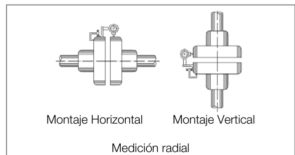
Figura 4.6: Alineación paralela
