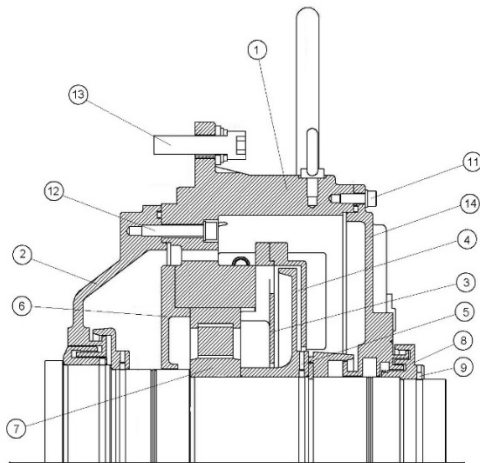
Figura 7.4: Partes del cojinete de rodamiento a aceite
