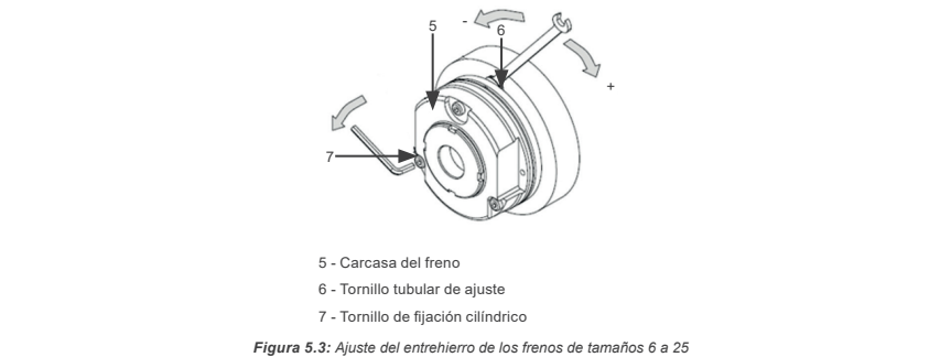
Figura 5.3: Ajuste del entrehierro de los frenos de tamaños 6 a 25
