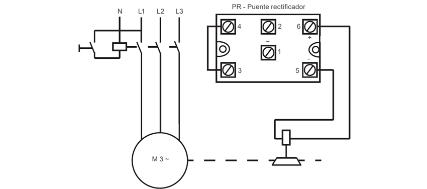
Figura 2.1: Esquema de conexión en el puente rectificador para frenado normal
