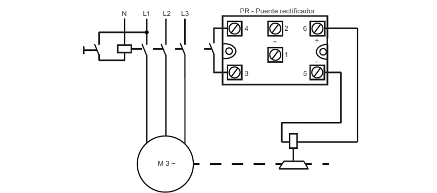
Figura 2.2: Esquema de conexión del puente rectificador para frenado rápido
