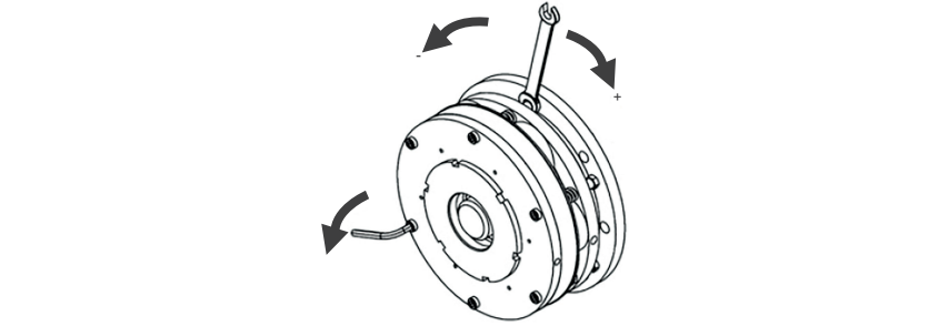
Figura 5.6: Ajuste del entrehierro en los frenos de tamaños 25 y 31
