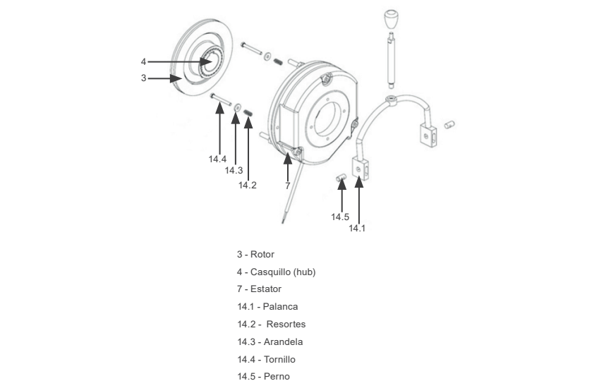
Figura 6.2: Componentes que hacen parte de la palanca de desbloqueo
