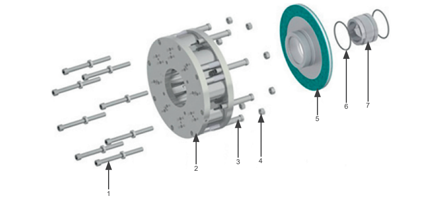
Figura 5.2: Componentes del freno electromagnético - tamaño 25 y 31 (800 a 2400 Nm)
