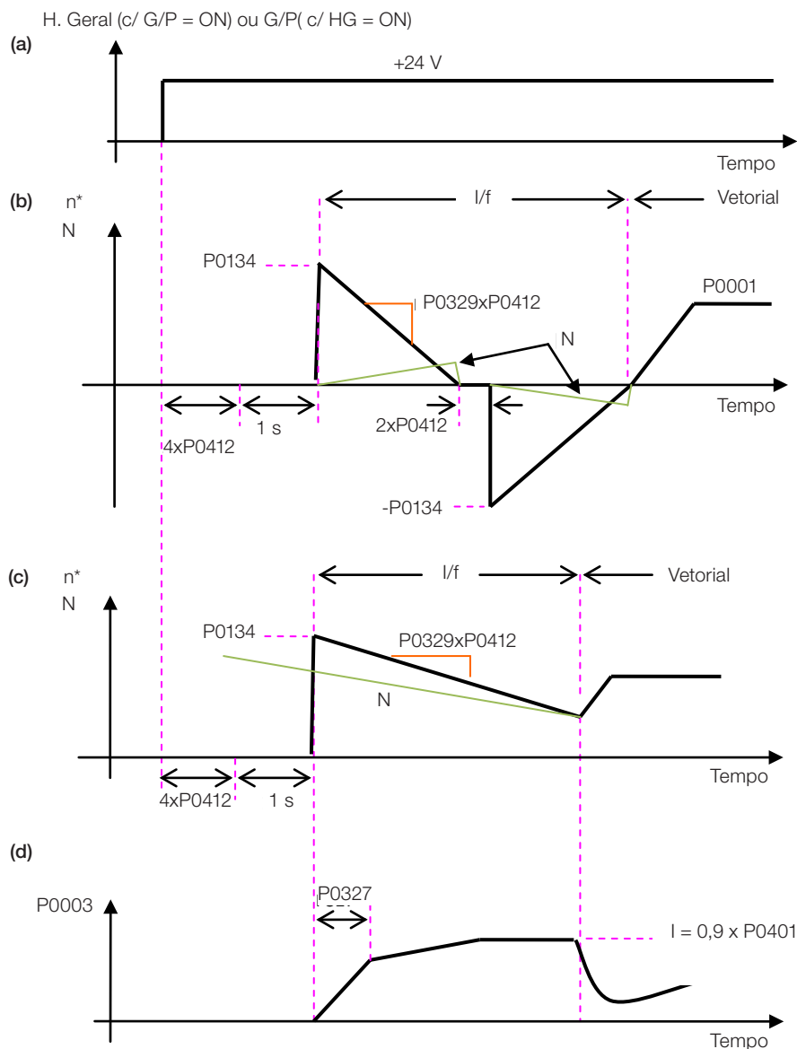
Figura 14.3: (a) a (d) Influência de P0327 e P0329 durante o Flying Start (P0202 = 4)
