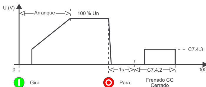
Figura 11.34: Frenado CC.
