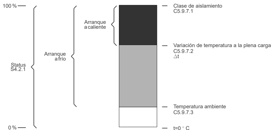
Figura 11.23: Rangos de temperatura del motor dentro de la clase de aislamiento.
