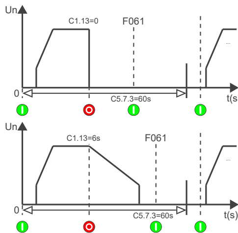
Figura 11.19: Tiempo entre arranques.
