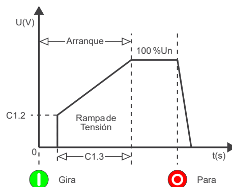
Figura 13.4: Arranque con Rampa de Tensión.
