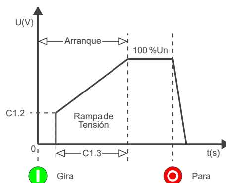
Figura 11.3: Rampa de aceleración por Rampa de Tensión.
