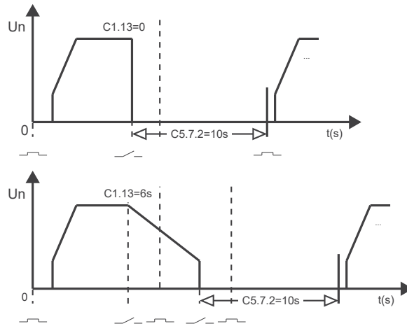
Figura 11.18: Accionamiento vía entrada digital (DI1).
