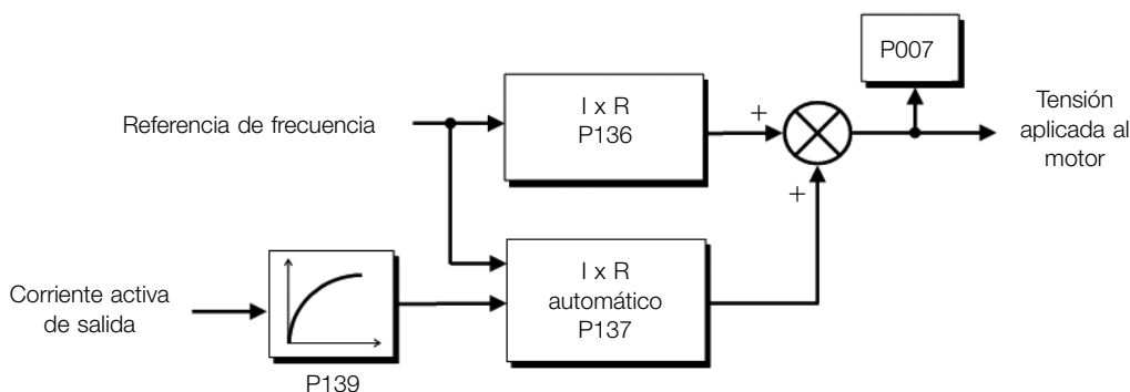
Figura 8.16: Diagrama de bloques del boost de torque automático
