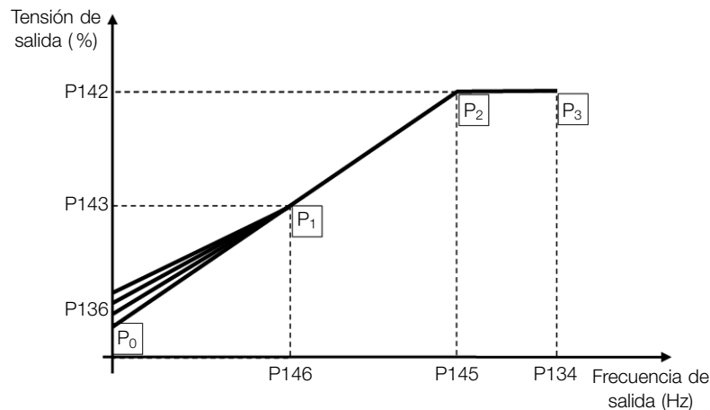
Figura 8.14: Región del boost de torque para modo del control V/f
