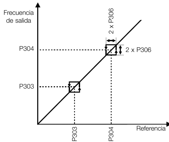
Figura 8.10: Actuación de la frecuencia evitada
