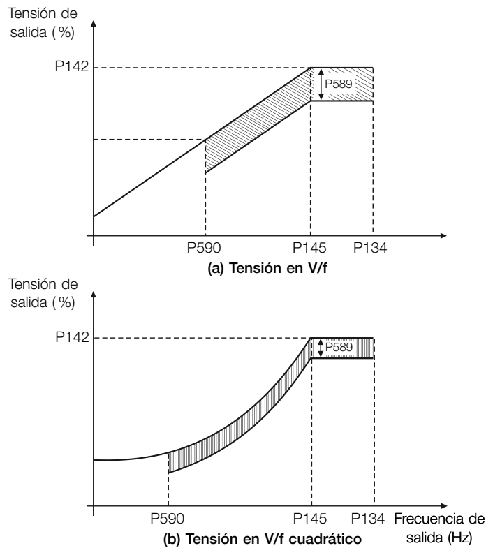
Figura 8.18: (a) y (b) Ejemplo de comportamiento de la tensión en V/f y V/f cuadrático
