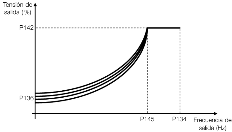
Figura 8.15: Región del boost de torque para modo del control V/f Cuadrático
