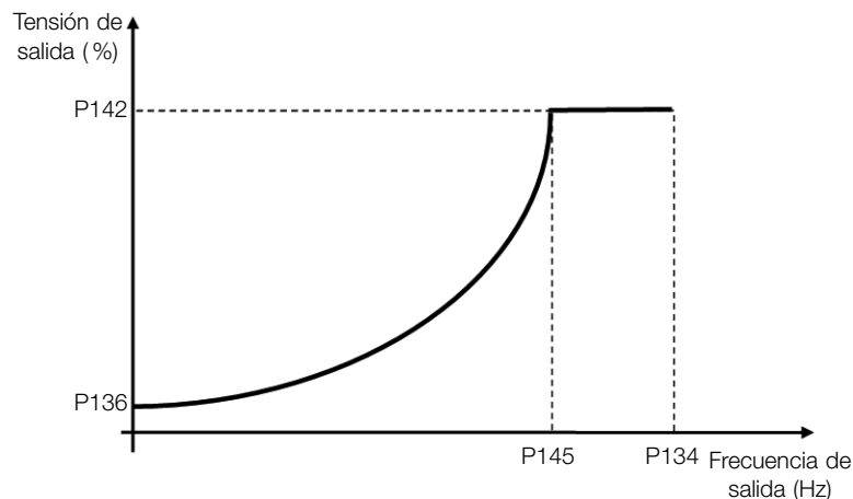
Figura 8.13: Curva V/f Cuadrática
