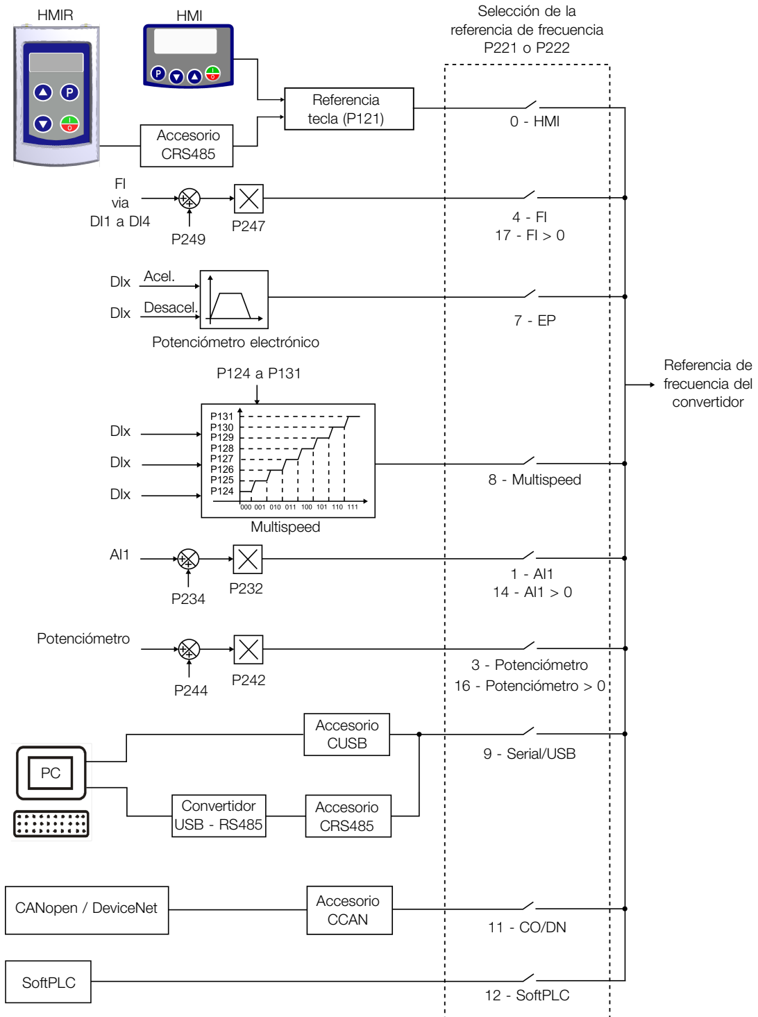
Figura 7.2: Estructura de selección de la referencia de frecuencia
