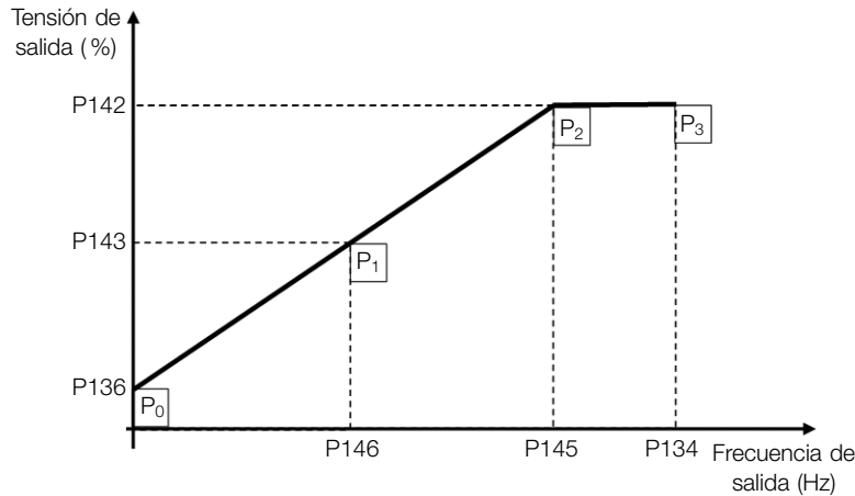
Figura 8.12: Curva V/f
