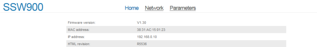
Figura 8.1: Página WEB
