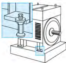
Рисунок 4.9. Анкерные болты
