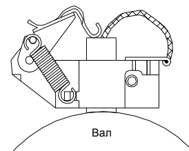
Рисунок 7.1. Щетка заземления вала
