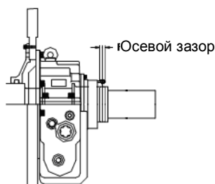
Рисунок 4.16. Метка магнитного центра
