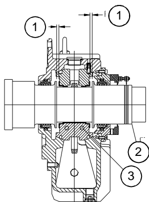
Рисунок 4.15. Подшипник скольжения
