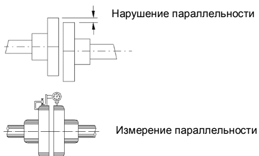
Рисунок 4.10. Регулировка соосности
