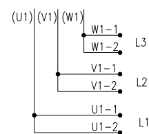
Рисунок 4.5. Параллельные соединения
