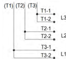
Рисунок 4.6. Параллельные соединения
