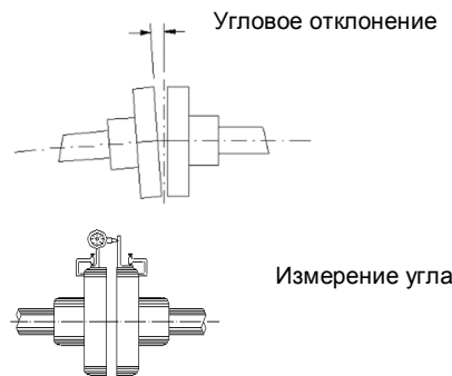
Рисунок 4.11. Угловое выравнивание
