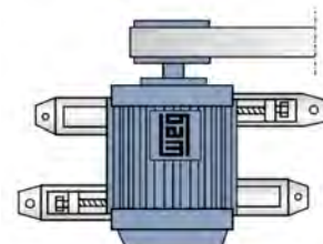
Рисунок 4.8. Скользящее основание
