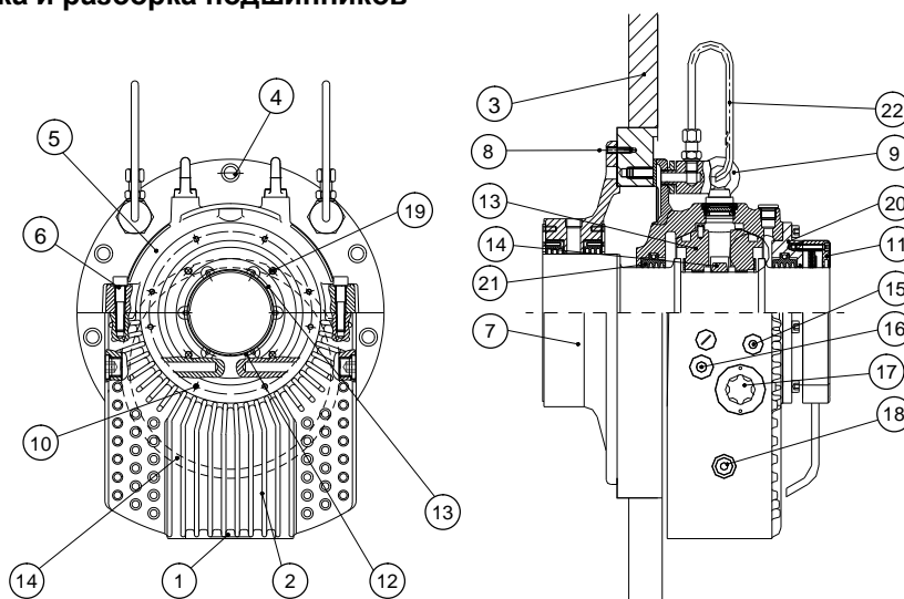
Рисунок 7.6. Компоненты подшипника скольжения
