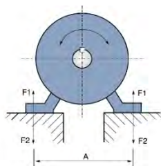
Рисунок 4.7. Нагрузка на основание
