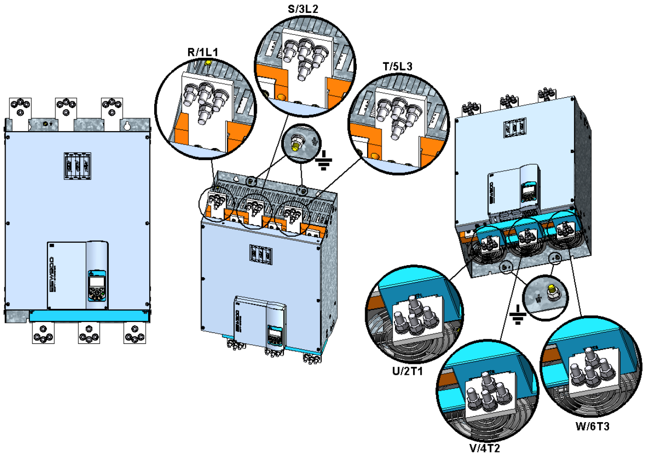
Figura 3.10: Borne de potencia y puesta a tierra, mecánica G
