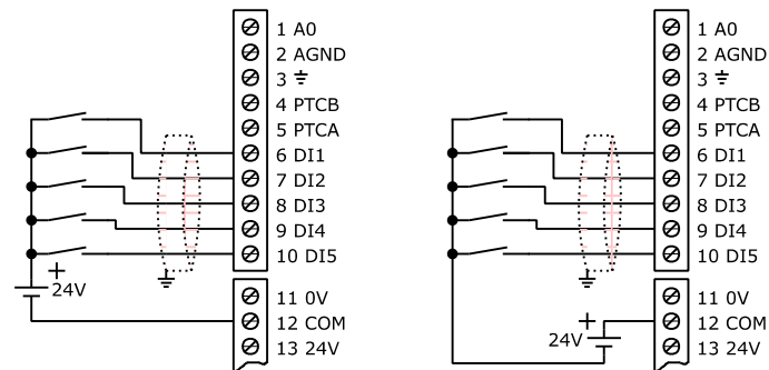
Figura 3.19: Esquema de conexión de las entradas digitales utilizando fuente externa
