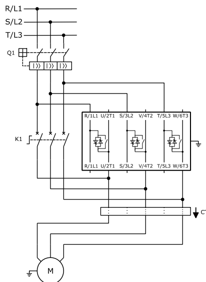
Figura 8.9: Esquema de conexión del contactor externo
