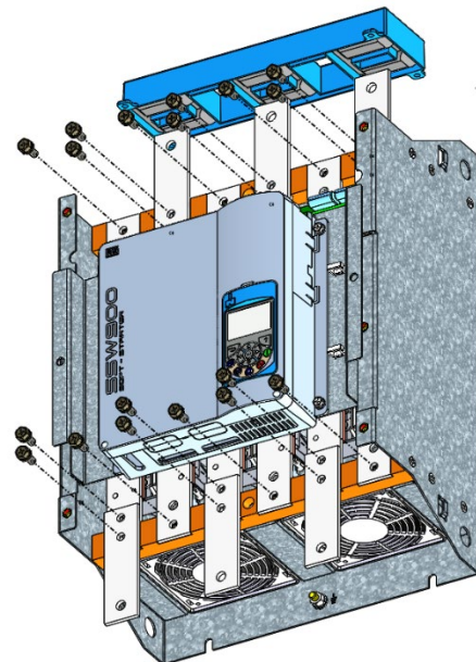
Figura 8.6: Colocando los barramientos y CT
