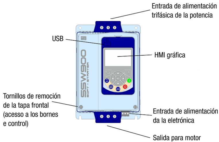
Figura 2.1: Vista frontal del SSW900
