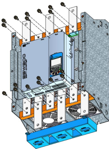
Figura 8.5: Retirando los barramientos y CT
