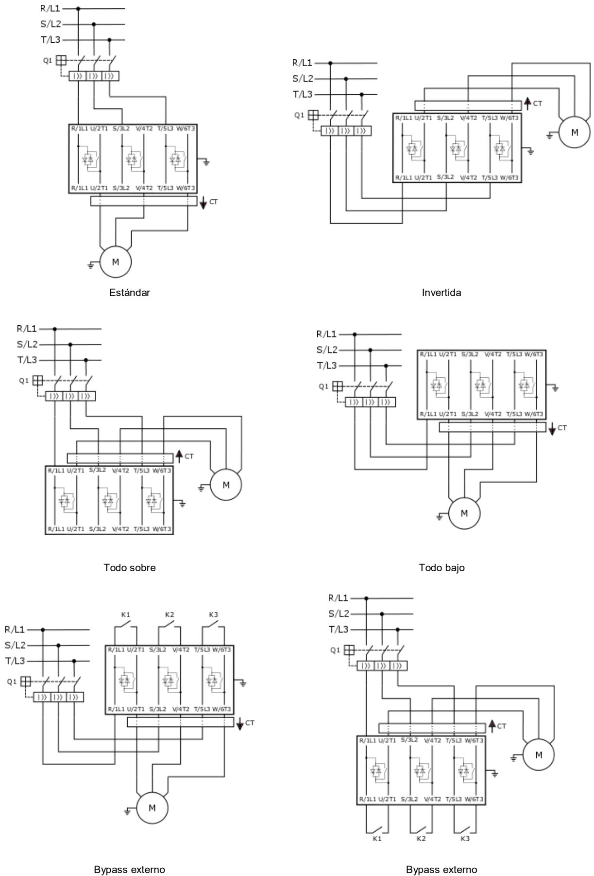
Figura 8.1: Conexión estándar de la mecánica E al motor con tres cables
