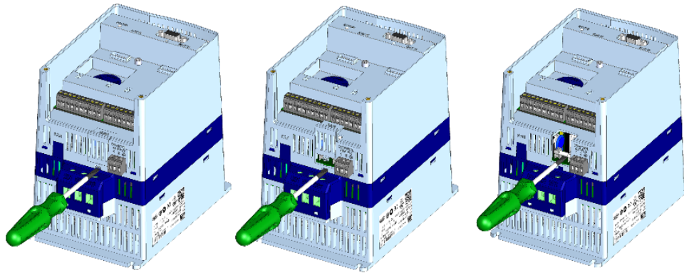
Figura 5.1: Procedimiento para cambio del fusible de la alimentación de la electrónica
