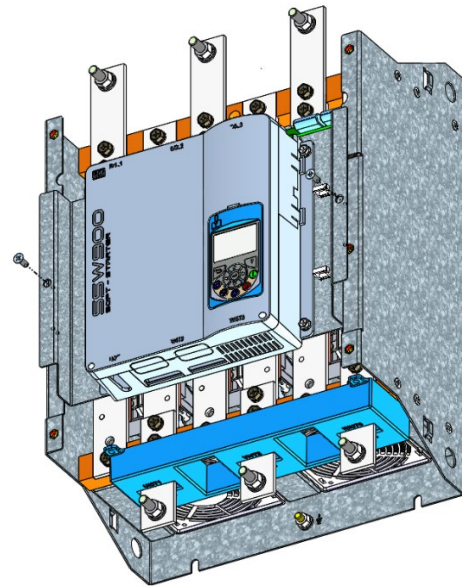
Figura 8.4: Moviendo el control
