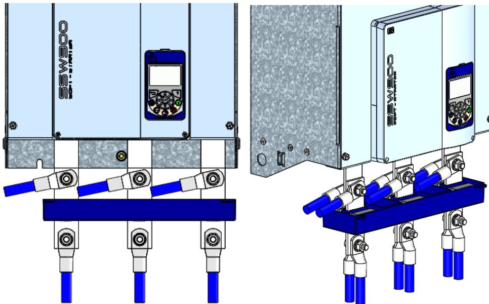
Figura 8.10: Sugerencia de salida de cable
