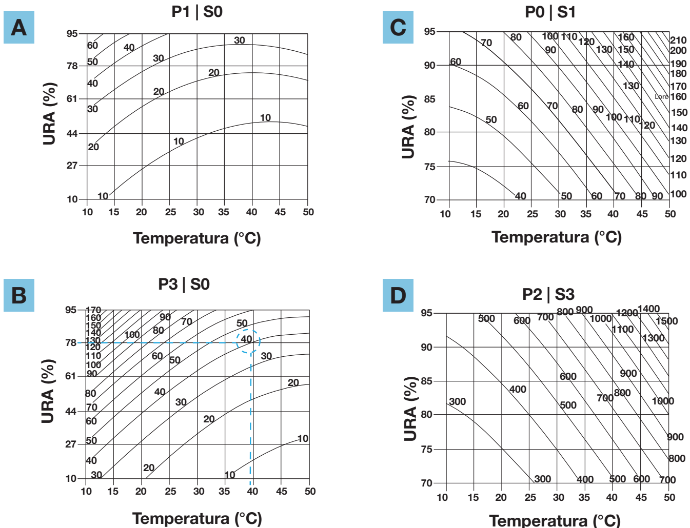
Figura 1: Efeito das características ambientais e climáticas sobre o aço-carbono.
