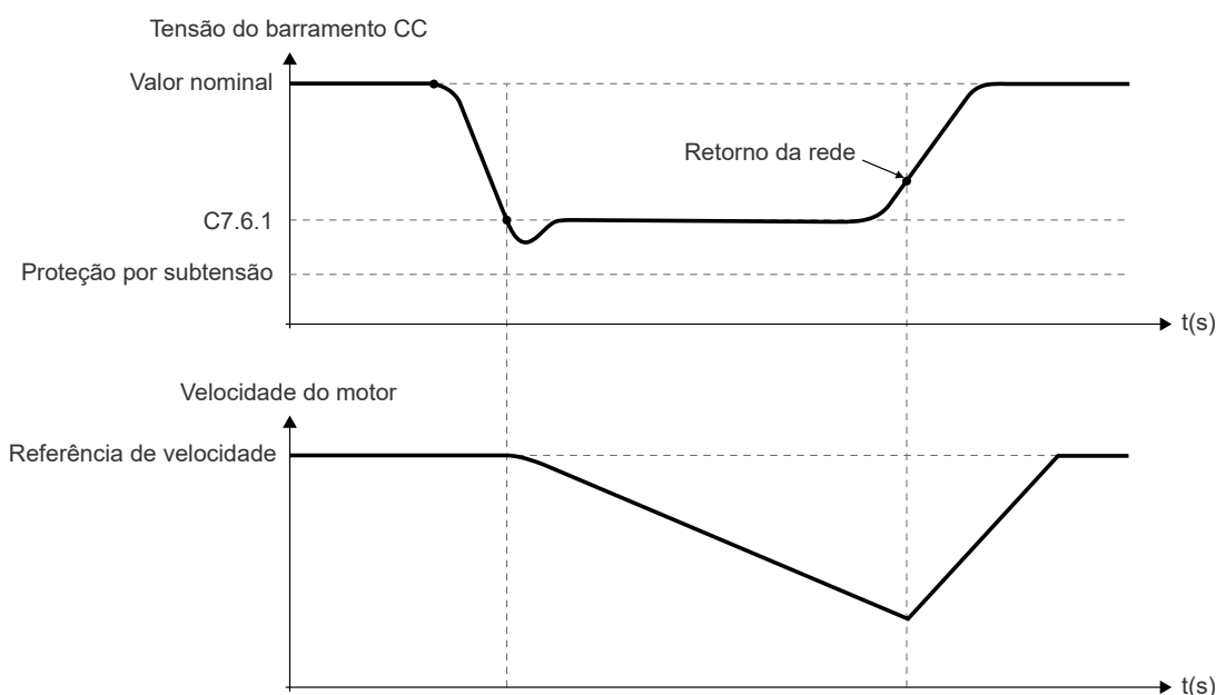
Figura 9.20: Esquema ilustrativo da operação da função Ride-Through
