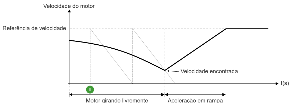
Figura 9.18: Esquema ilustrativo da função Flying Start
