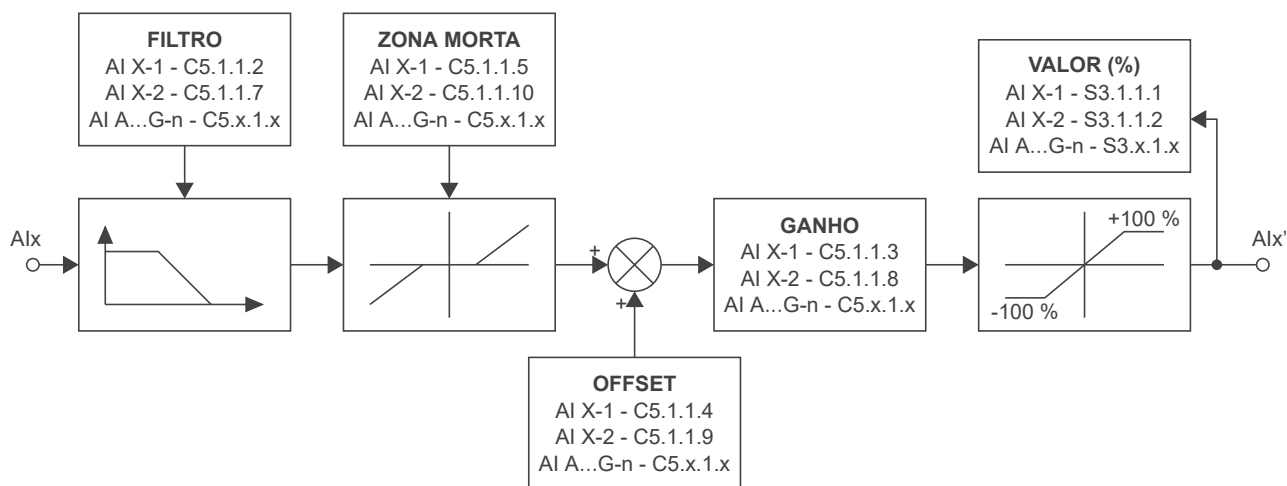
Figura 9.37: Diagrama de blocos da entrada analógica
