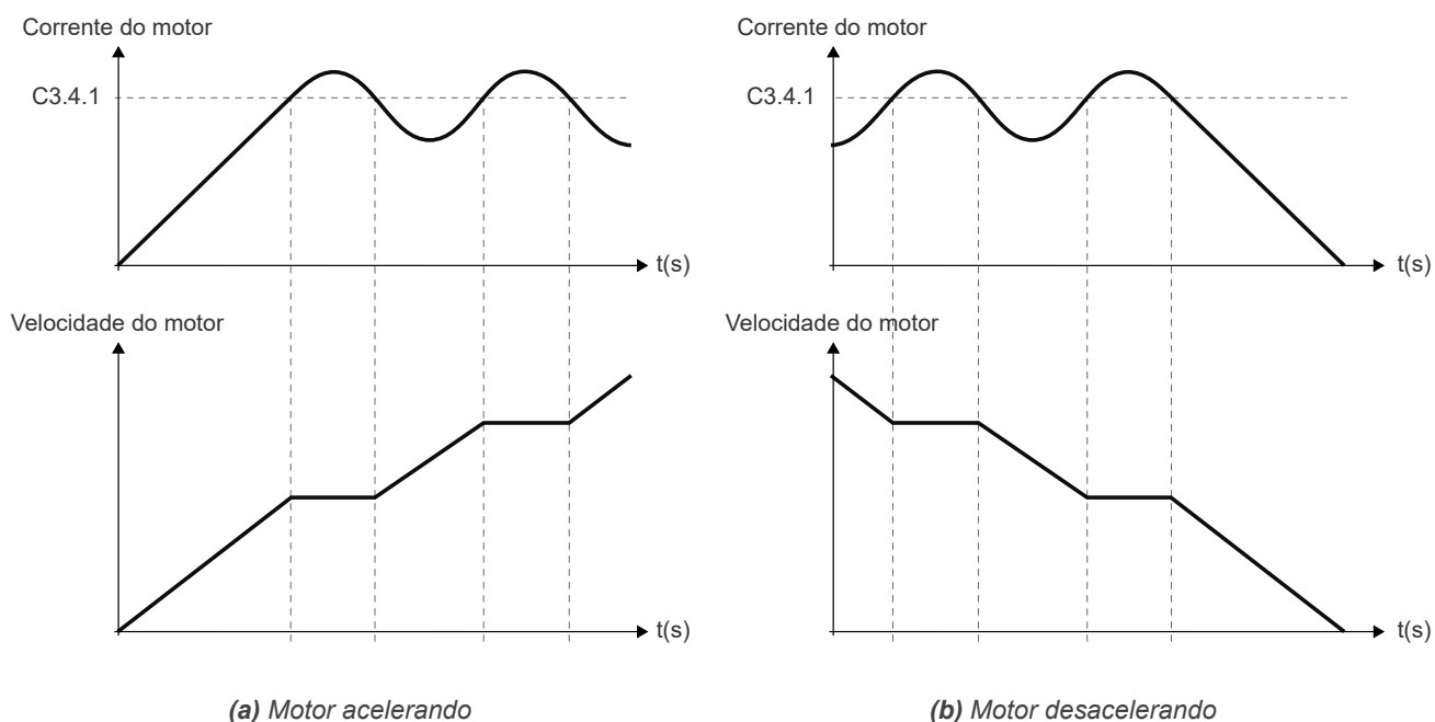
Figura 9.14: Limitação de corrente durante a aceleração e a desaceleração
