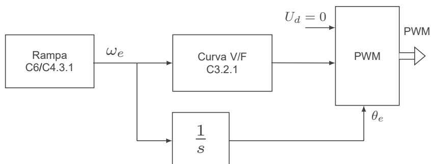
Figura 9.6: Diagrama de blocos do controle escalar para motor de indução
