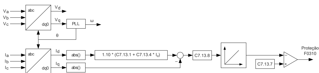
Figura 9.50: Esquema da proteção do secundário do transformador de entrada
