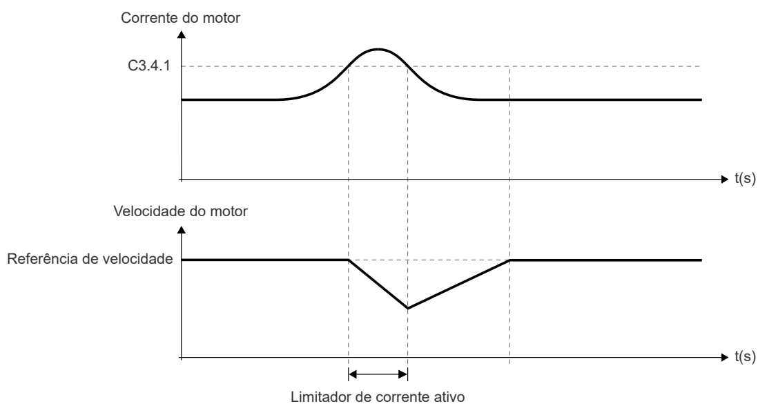
Figura 9.15: Limitação de corrente com o motor operando em velocidade constante
