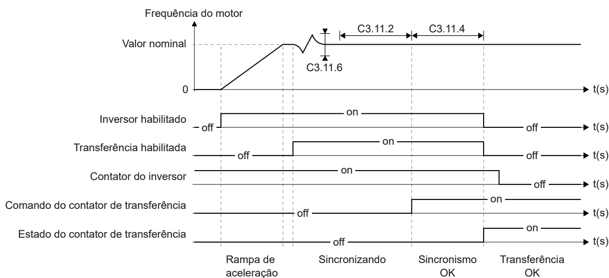
Figura 9.23: Diagrama de operação da função de transferência síncrona
