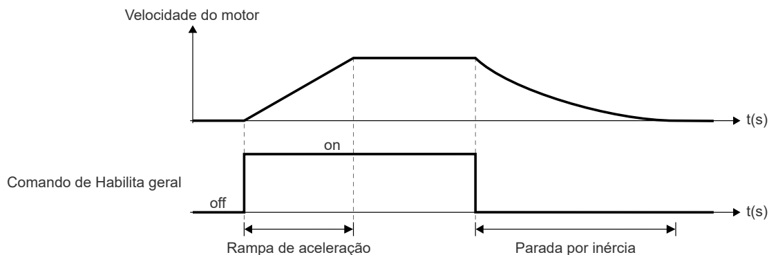
Figura 9.24: Atuação do comando habilita geral
