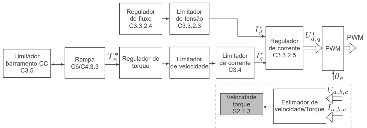
Figura 9.10: Diagrama de bloco do controle vetorial do motor de indução no modo torque
