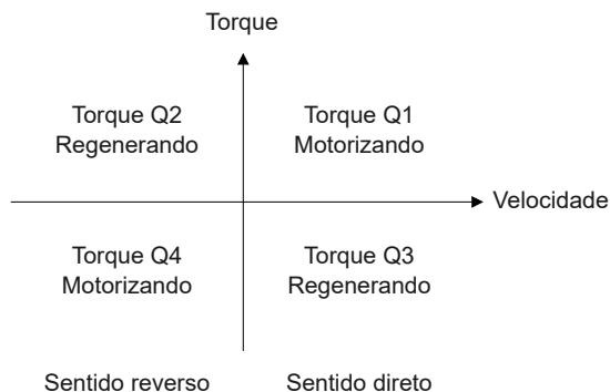
Figura 9.12: Convenção dos limitadores de torque do motor nos quatro quadrantes de operação
