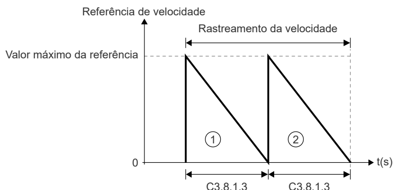
Figura 9.19: Esquema ilustrativo da identificação da velocidade do rotor pela função Flying Start
