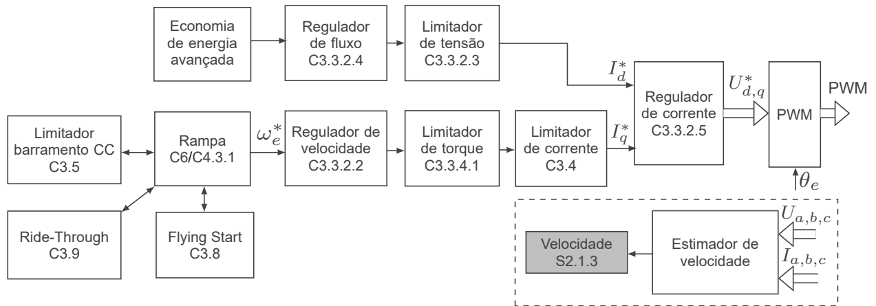
Figura 9.9: Diagrama de bloco do controle vetorial do motor de indução no modo velocidade
