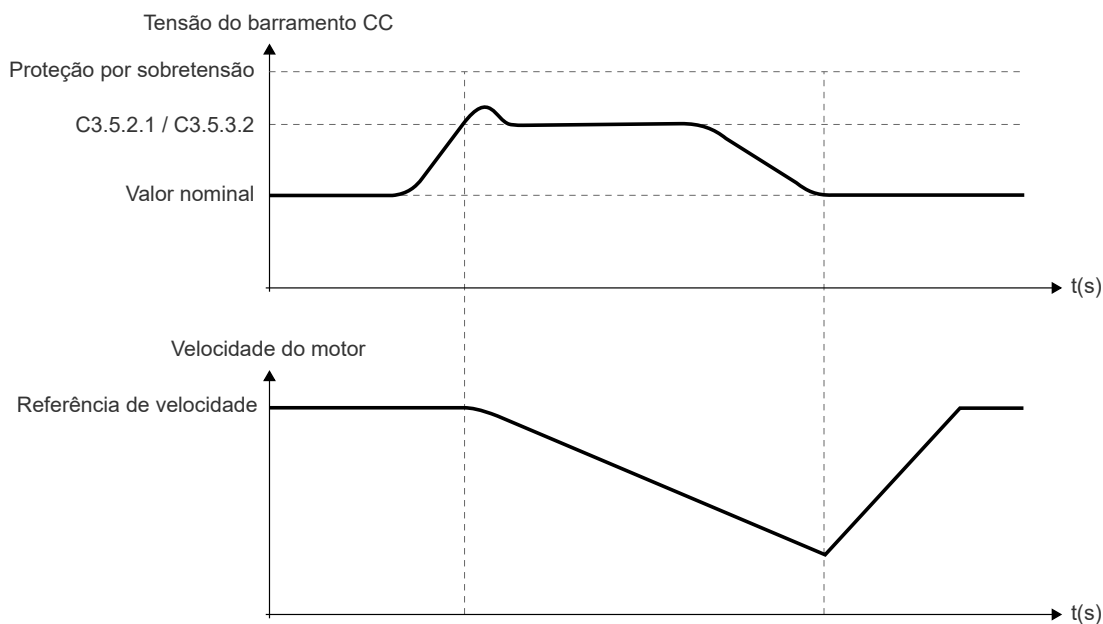
Figura 9.17: Limitação do barramento CC quando o motor está operando com velocidade constante
