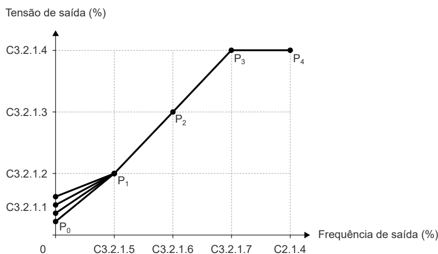
Figura 9.7: Região do boost de torque
