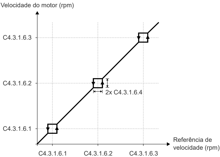
Figura 9.35: Curva de atuação das “Velocidades Evitadas”
