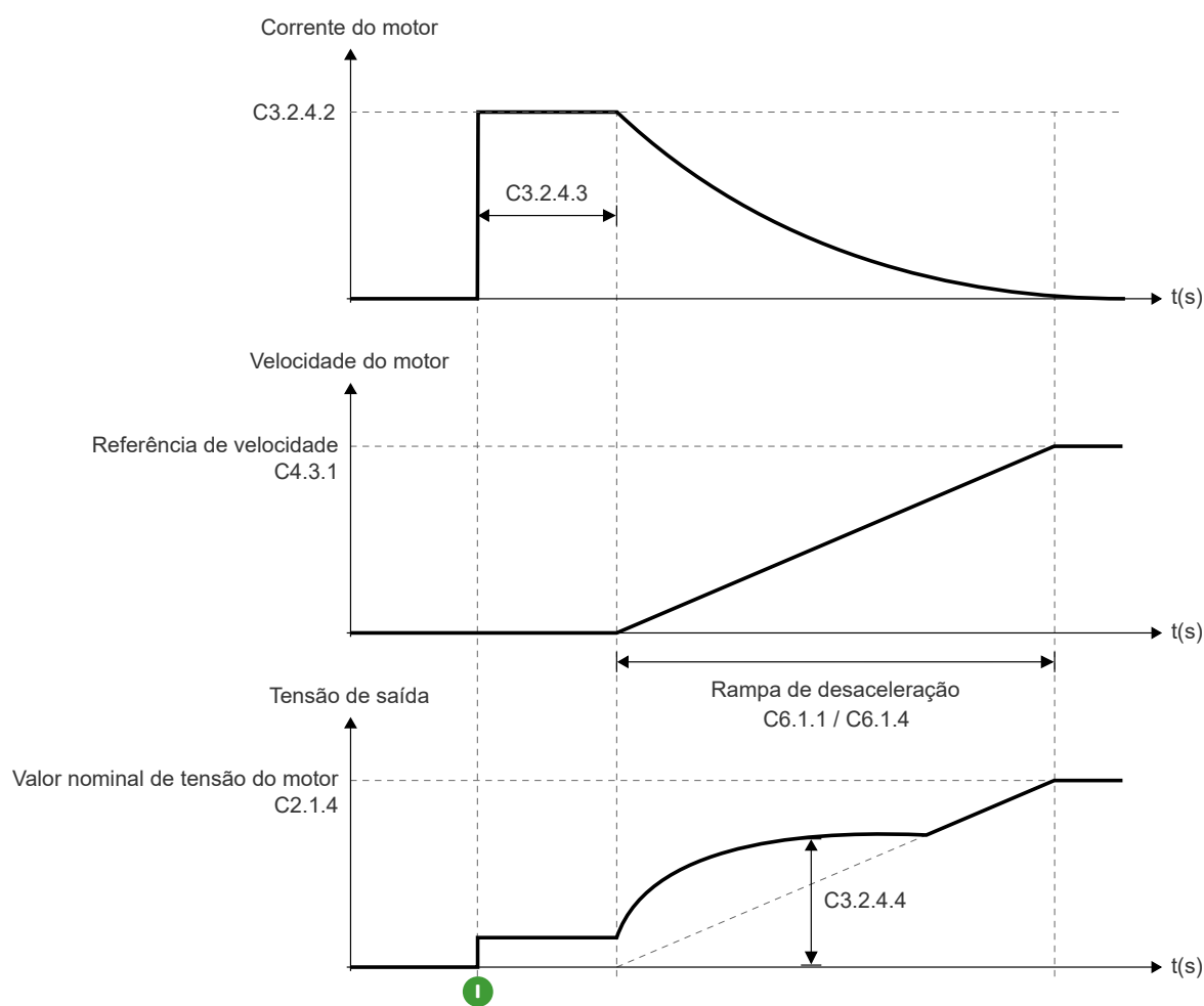
Figura 9.8: Esquema ilustrativo da operação da função pré-magnetização
