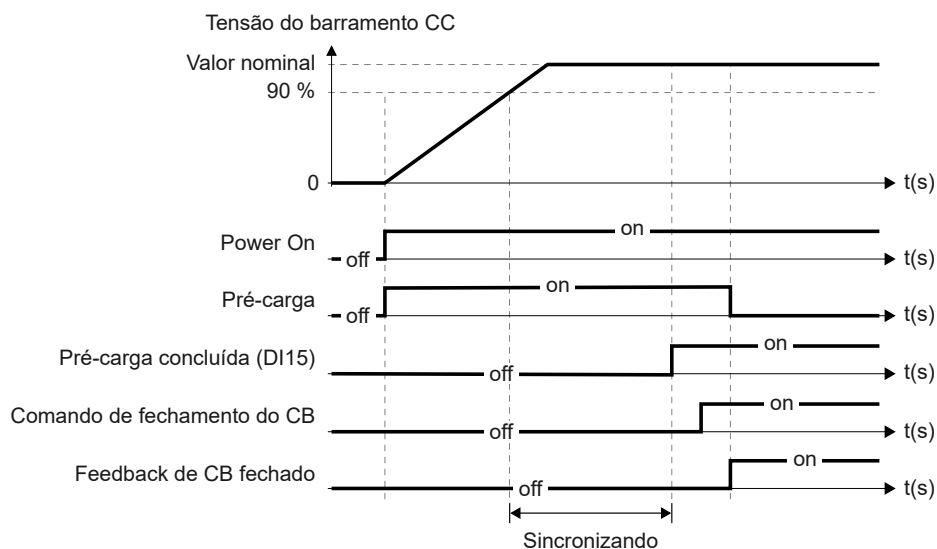
Figura 9.5: Pré-carga síncrona
