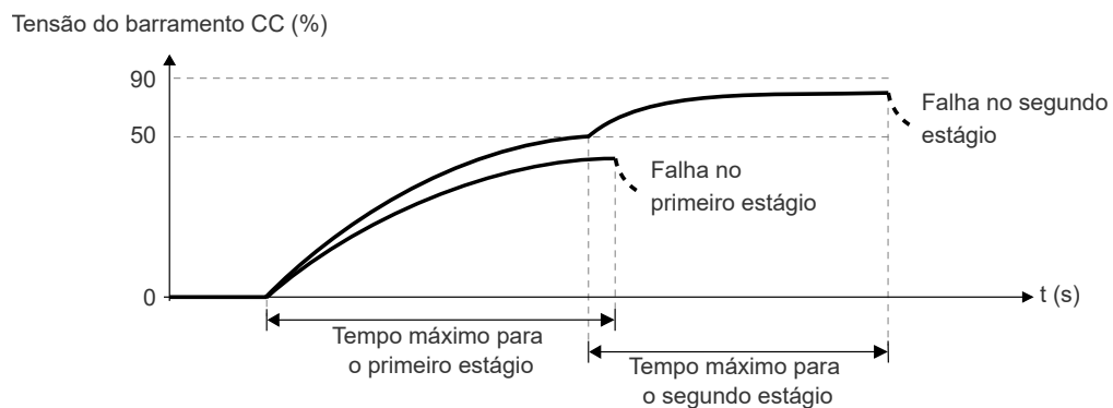
Figura 9.3: Exemplo de time-out na pré-carga
