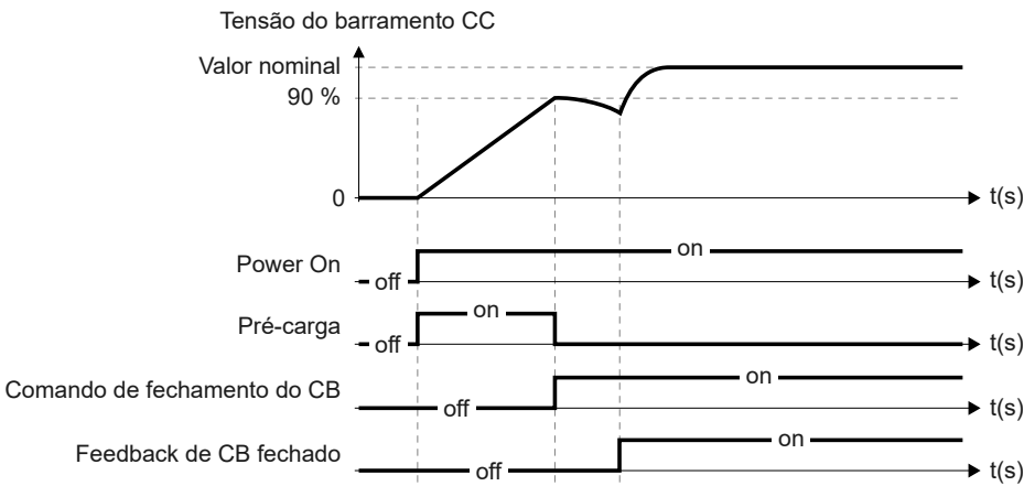
Figura 9.4: Pré-carga padrão
