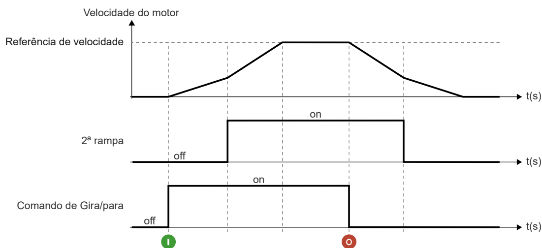
Figura 9.46: Atuação do comando 1ª/2ª rampa
