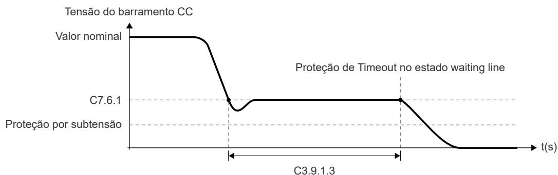
Figura 9.21: Time-out no retorno da rede
