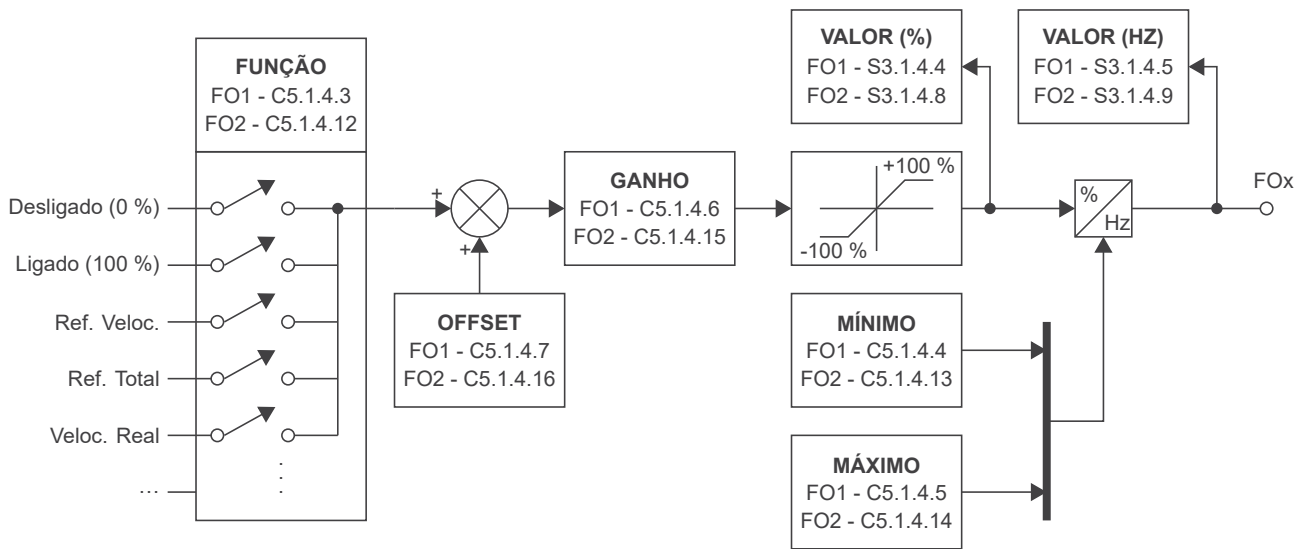
Figura 9.42: Diagrama de blocos da saída em frequência
