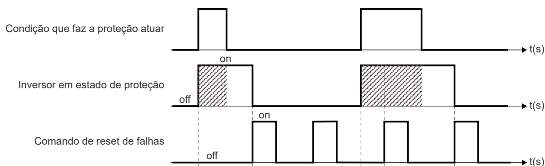
Figura 9.32: Atuação do comando Reset de Falha/Proteção
