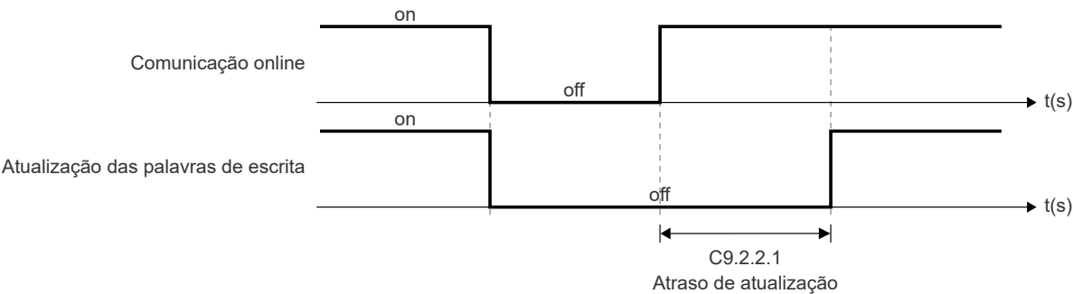
Figura 9.51: Atraso na atualização das palavras de I/O
