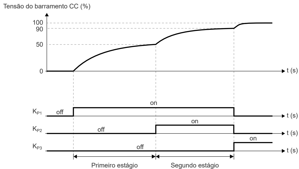
Figura 9.2: Estágios da pré-carga
