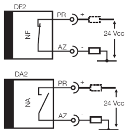
Figura 1: Diagrama elétrico
