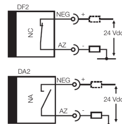
Figura 1: Diagrama eléctrico
