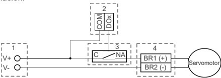
Figura 9.3: Conexión del freno electromagnético
