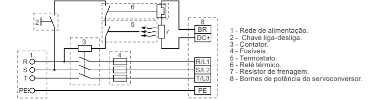
Figura 9.1: Conexões de potência e aterramento
