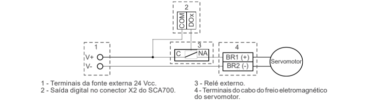
Figura 9.3: Conexão do freio eletromagnético
