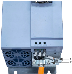
Figura 9.2: Conexiones de salida y puesta a tierra del motor
