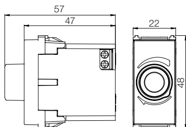
Módulo dimmer
