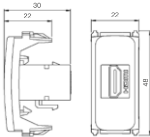
Tomada HDMI
