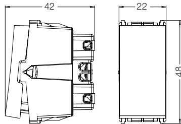
Interruptor paralelo
