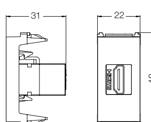
Módulo HDMI
