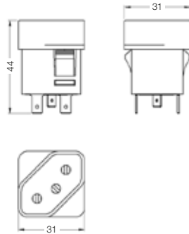
Tomada de painel quadrada colar externo (faston)
