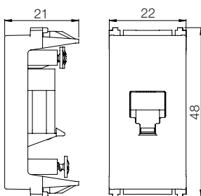
Módulo RJ11
