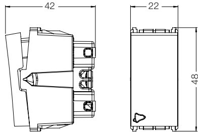
Pulsador campainha
