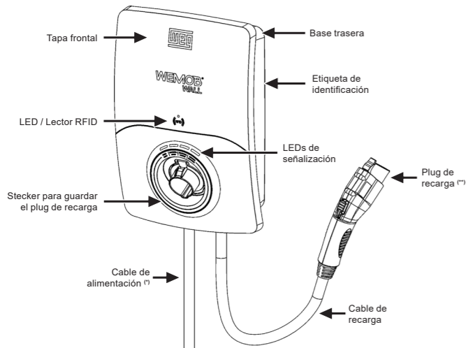
Figura 2.1: Visión general de la WEMOB-WALL
