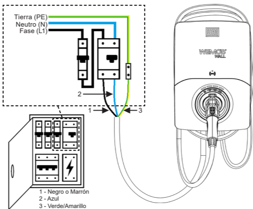
(a) Con disyuntor monofásico y DR
