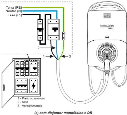
(a) com disjuntor monofásico e DR
