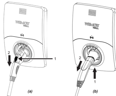
Figura 5.4: (a) e (b) Procedimento para retirada do plugue do soquete nas estações de recarga com cabos tipo 1 e NACS
