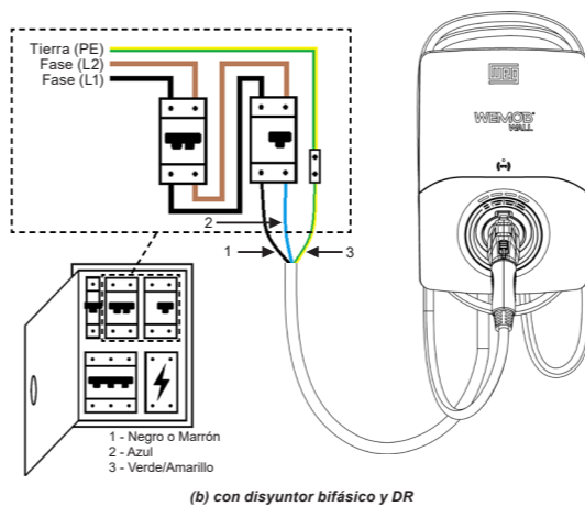
Figura 5.3: (a) y (b) ejemplos de conexión eléctrica monofásica (L1-N-PE) y bifásica (L1-L2-PE)
