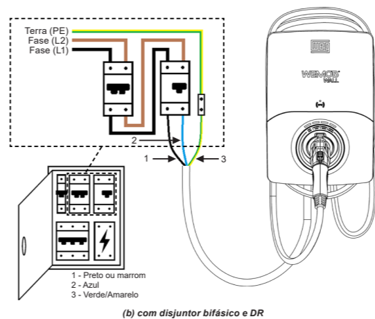
(b) com disjuntor bifásico e DR
