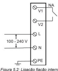
Figura 5.2: Ligação fiação interna
