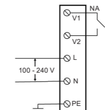
Figura 5.2: Conexión eléctrica interna
