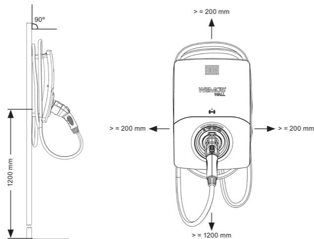
Figura 4.1: Posición de montaje y distanciamiento de la WEMOB-WALL
