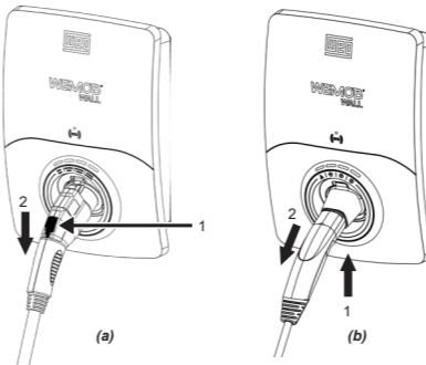
Figura 5.4: (a) y (b) Procedimiento para retirada del plug del stecker en las estaciones de recarga con cables tipo 1 y NACS
