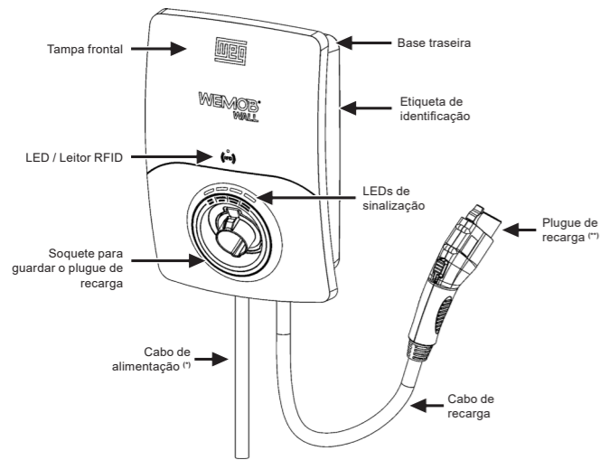
Figura 2.1: Visão geral da WEMOB-WALL
