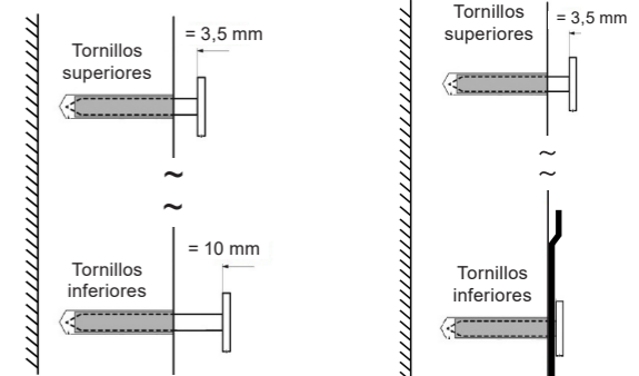
(a) Fijación sin el soporte metálico
