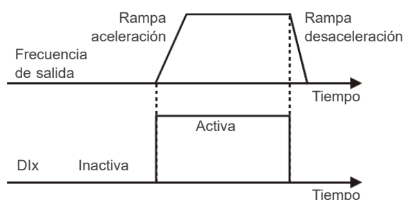
Figura 9.6: Ejemplo de la función Gira/Para
