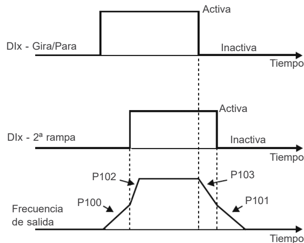
Figura 9.14: Ejemplo de la función 2ª Rampa
