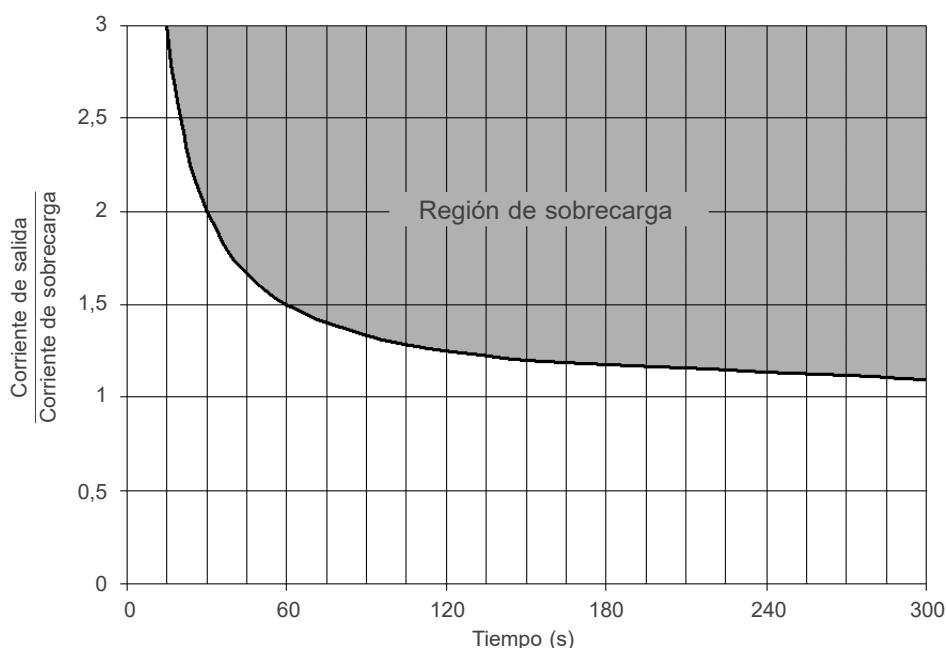
Figura 10.2: Actuación de la sobrecarga del motor
