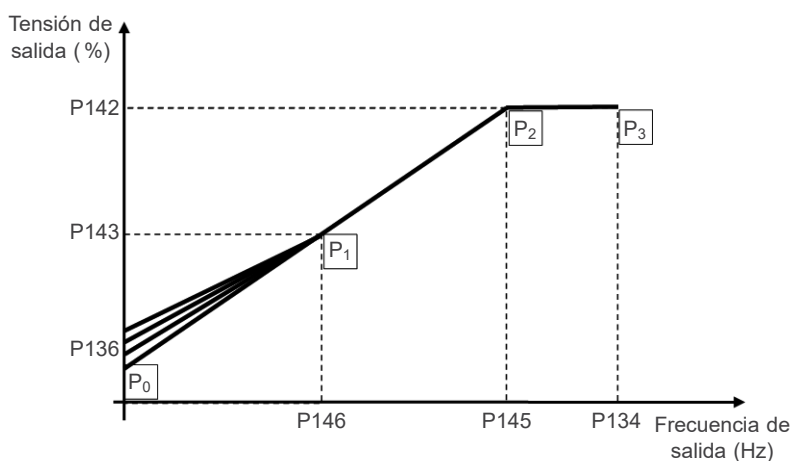
Figura 8.15: Región del boost de torque para modo de control V/f
