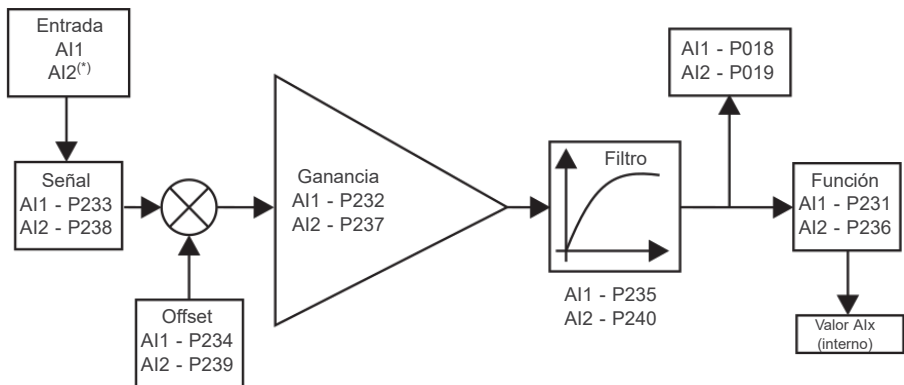
Figura 9.1: Diagrama de bloque de la entrada analógica (Alx)
