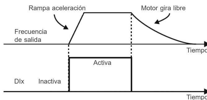
Figura 9.7: Ejemplo de la función Habilita General
