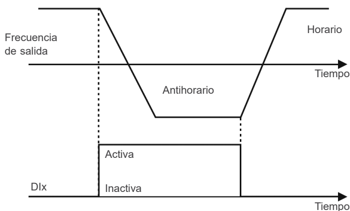
Figura 9.11: Ejemplo de la función Sentido de Giro
