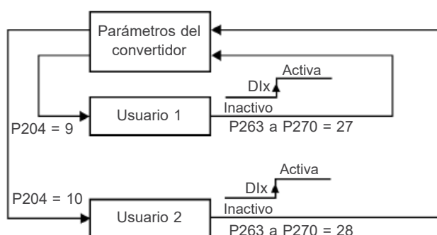
Figura 9.15: El diagrama de bloques de funciones carga al usuario 1 y al usuario 2
