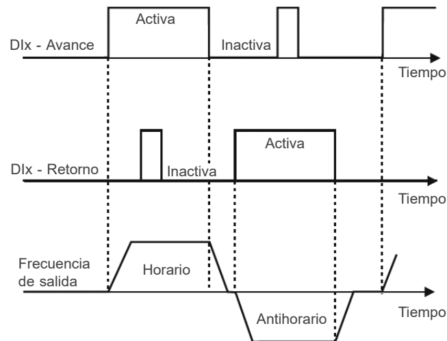
Figura 9.9: Ejemplo de la función Avance/Retorno
