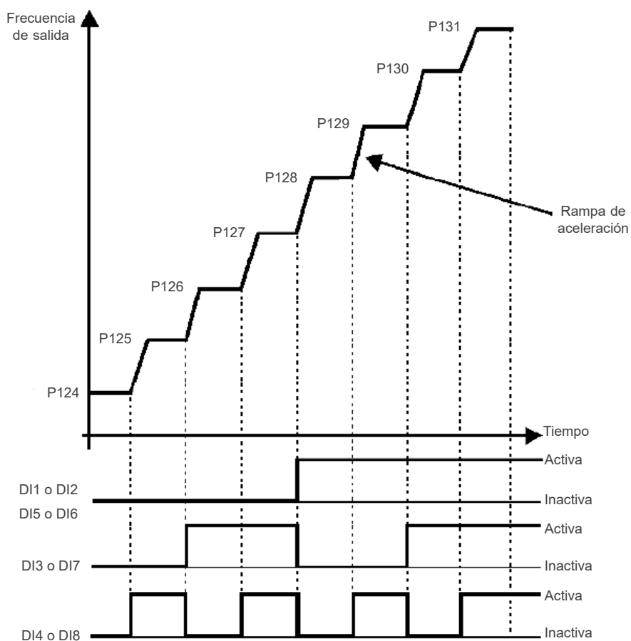
Figura 7.3: Gráfico de funcionamiento de la función Multispeed
