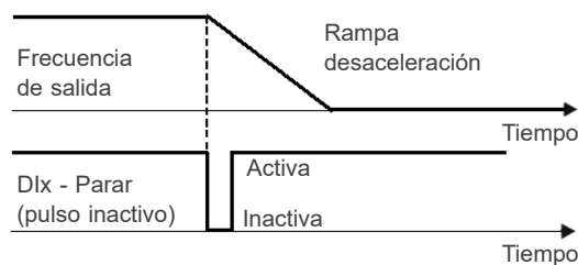
Figura 9.18: Ejemplo de función Stop con impulso inactivo
