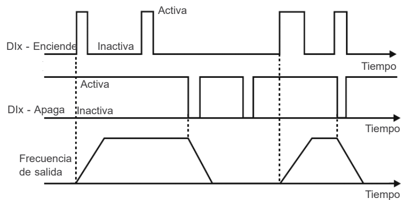
Figura 9.10: Ejemplo de la función Start/Stop
