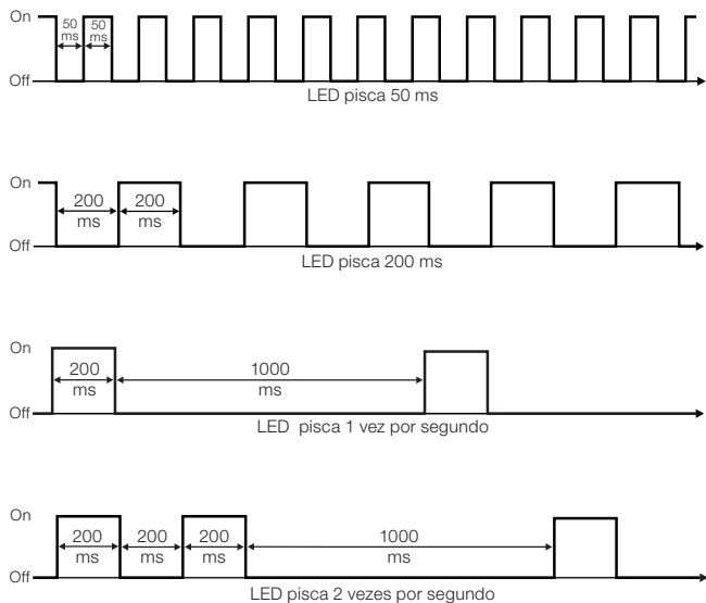
Figura 6.2: Diagrama de tempo para o comportamento da sinalização
