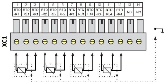
Figura 4.3: Esquema de ligação dos RTDs
