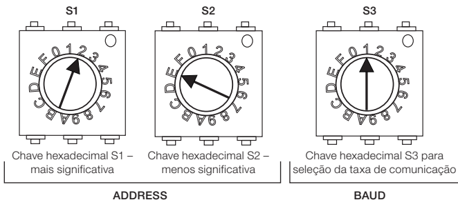
Figura 5.2: Chaves hexadecimais para configuração da RUW-05
