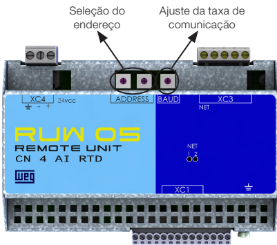
Figura 5.1: Chaves hexadecimal para configuração da RUW-05
