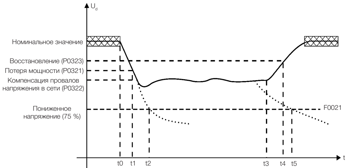
Рисунок 14.4: Запуск функции компенсации провалов напряжения в сети в векторном режиме
