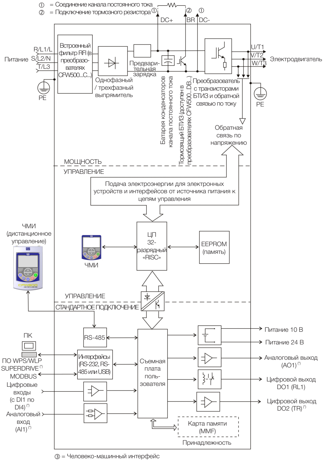
Рисунок 3.1: Блок-схема CFW500
