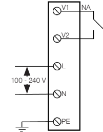
Figura 5.2: Conexión eléctrica interna
