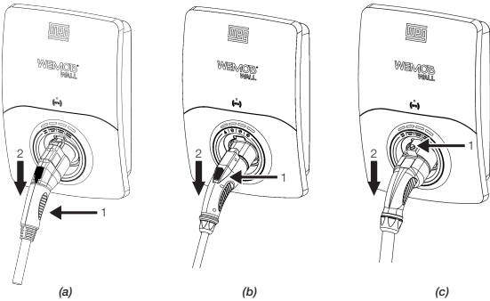
Figura 5.4: (a), (b) y (c) procedimiento para retrada del plug del stecker en las estaciones de recarga con cables tipo 1, GB/T y tipo 2
