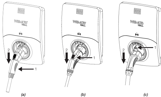
Figura 5.4: (a), (b) e (c) Procedimento para retirada do plugue do soquete nas estações de recarga com cabos tipo 1, GB/T e tipo 2
