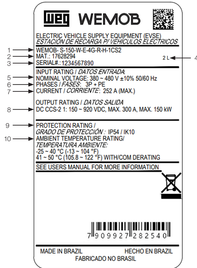
Figura 2.2: Etiqueta de identificação da WEMOB-STATION CCS
