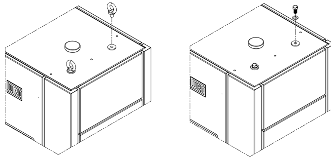
Figura 3.2: Detalhe de troca do olhal de içamento para parafuso, arruela e anel O'ring
