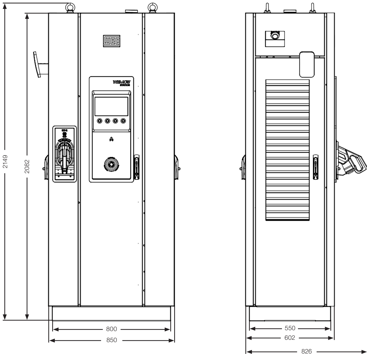
Figura 8.1: Dimensões da WEMOB-STATION em mm
