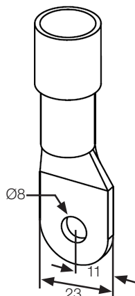
Figura 3.11: Especificação do terminal olhal - mm
