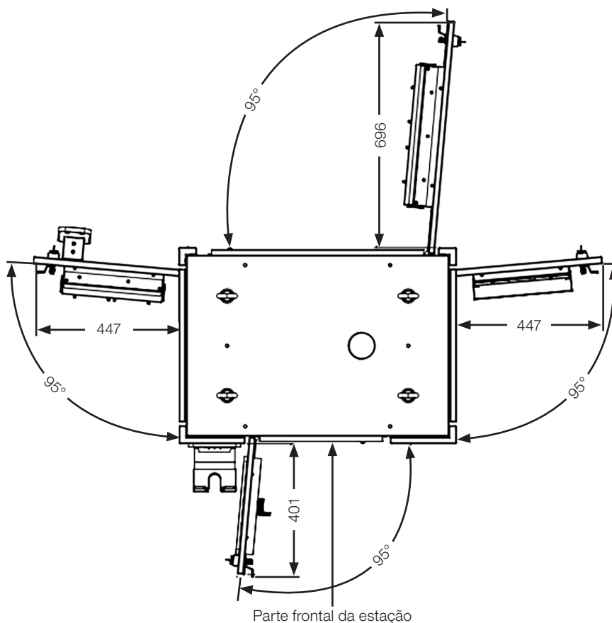
Figura 3.7: Área necessária para abertura completa das portas da estação - mm
