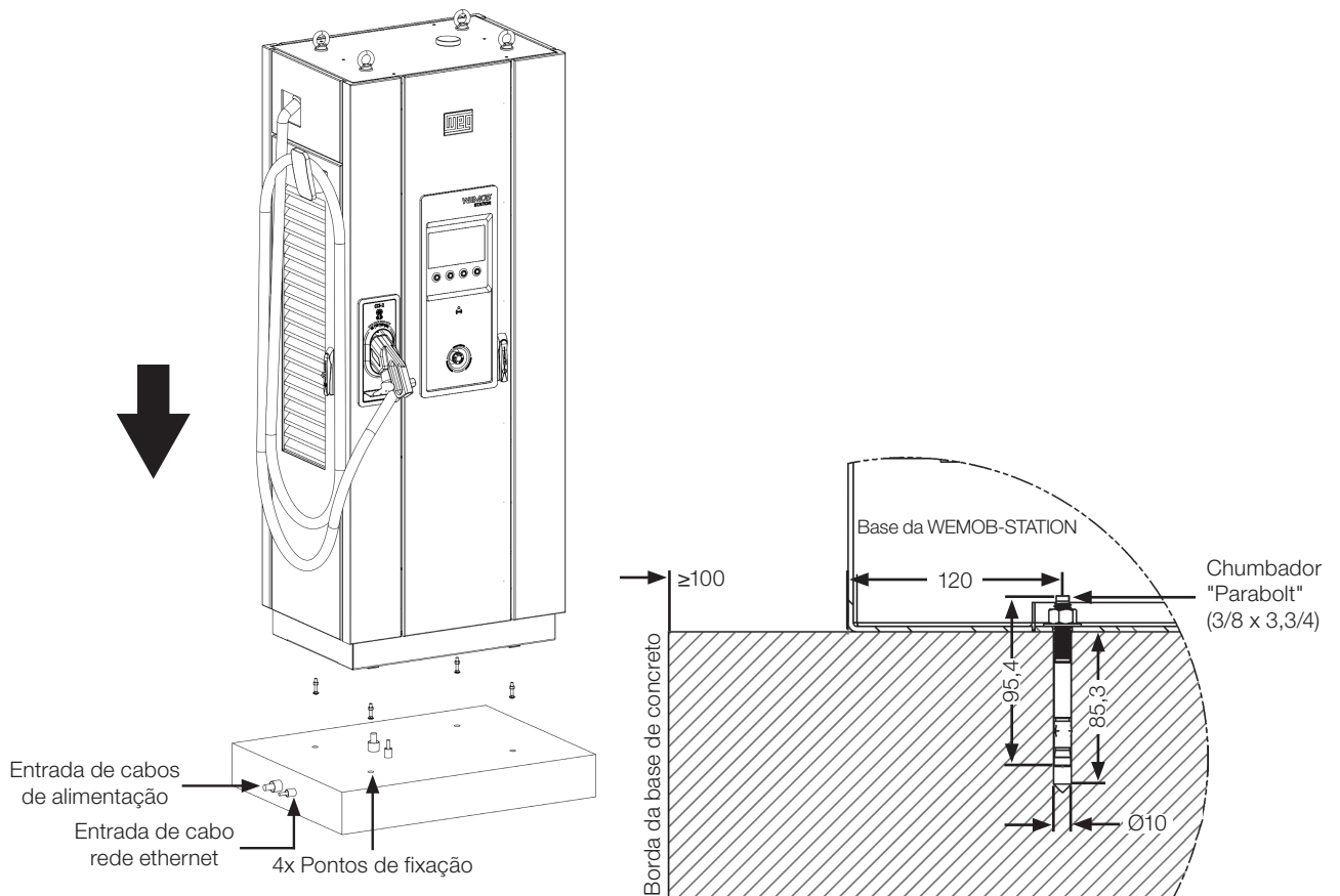
Figura 3.9: Detalhes dos pontos de fixação - mm
