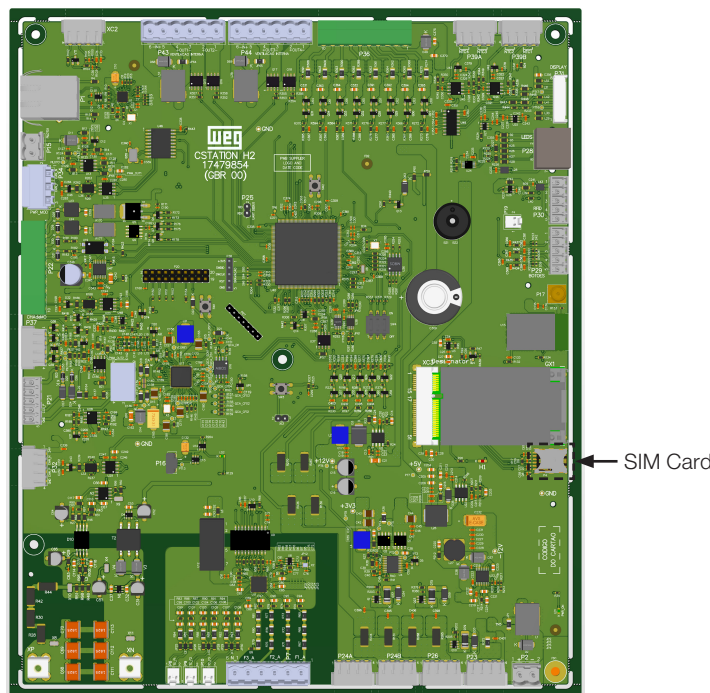
Figura 6.7: Localização do slot do SIM Card no cartão eletrônico de controle
