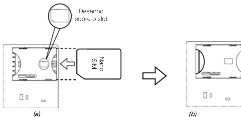
Figura 6.8: Procedimento para inserir o SIM Card
