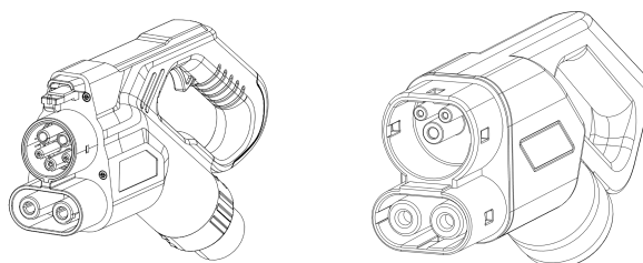
Figura 2.3: Modelo do conector da WEMOB-STATION CCS-1 e CCS-2
