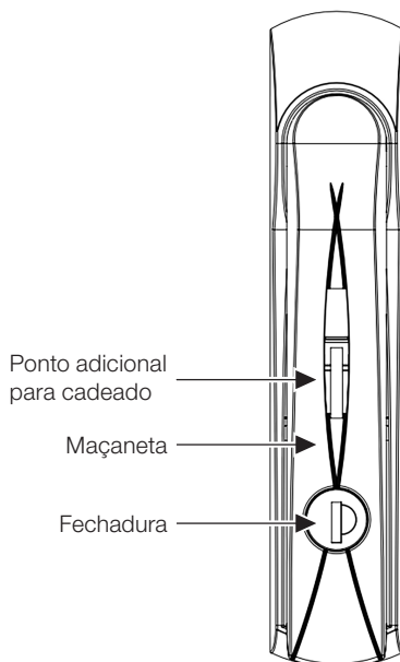
Figura 3.4: Fechadura localizada nas portas frontal/laterais/traseira
