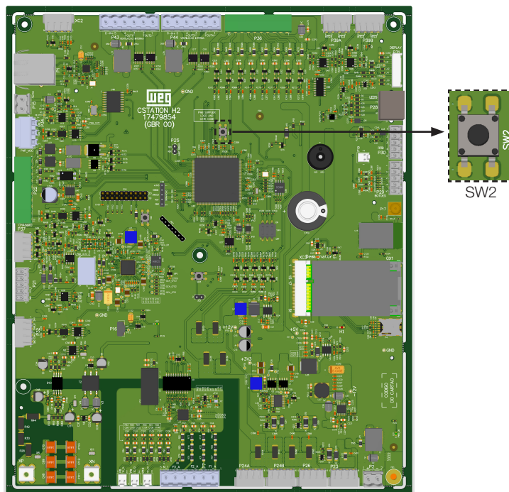
Figura 6.12: Localização do botão de reset "SW2" no cartão eletrônico
