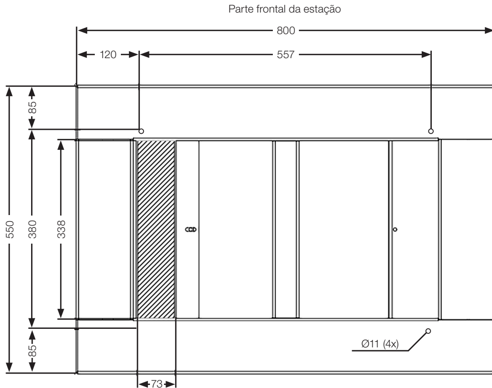
Figura 3.8: Dimensões para fixação e passagem dos eletrodutos da WEMOB-STATION - mm
