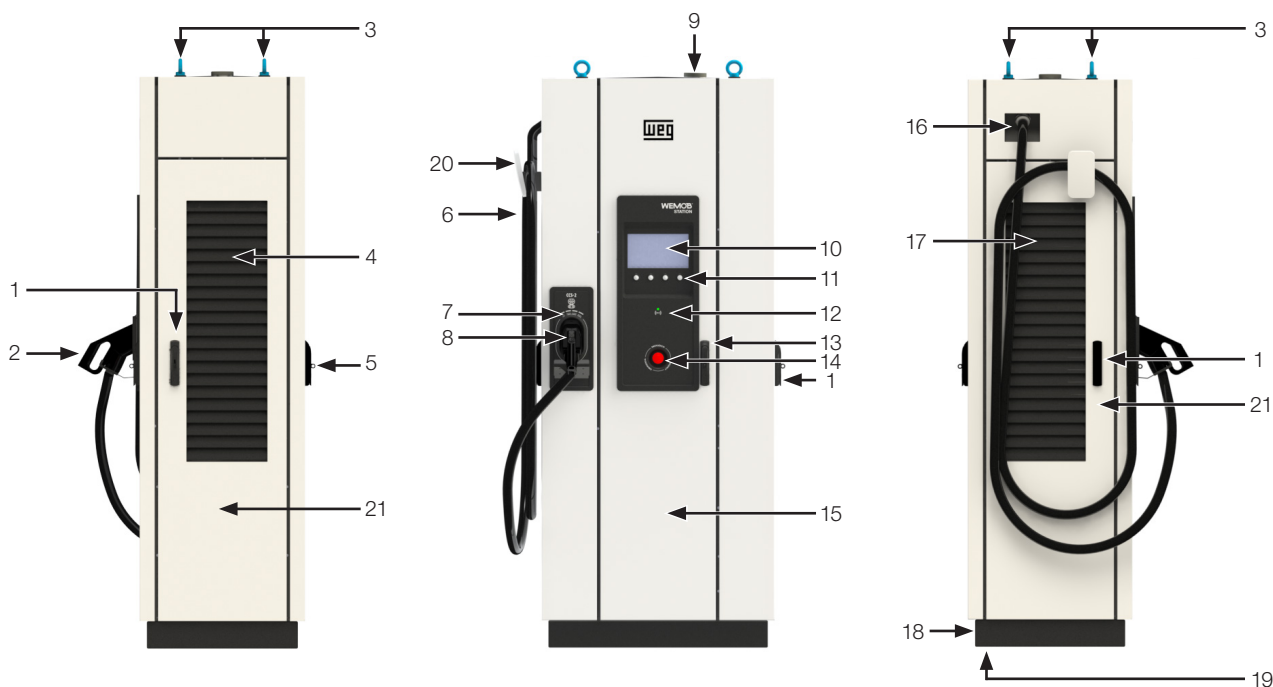
Figura 2.1: Visão geral da estação de Recarga WEMOB-STATION CCS
