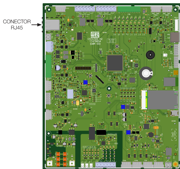
Figura 6.6: Localização do conector RJ45 no cartão eletrônico de controle
