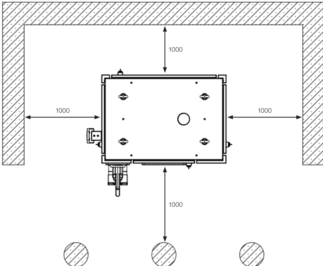
Figura 3.6: Distanciamento mínimo recomendado - mm
