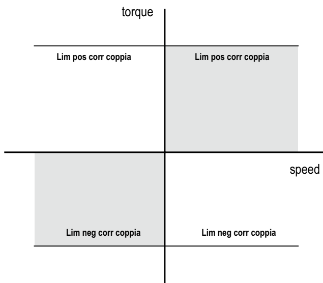
Limiti di coppia con Sel lim corr coppia = 1
