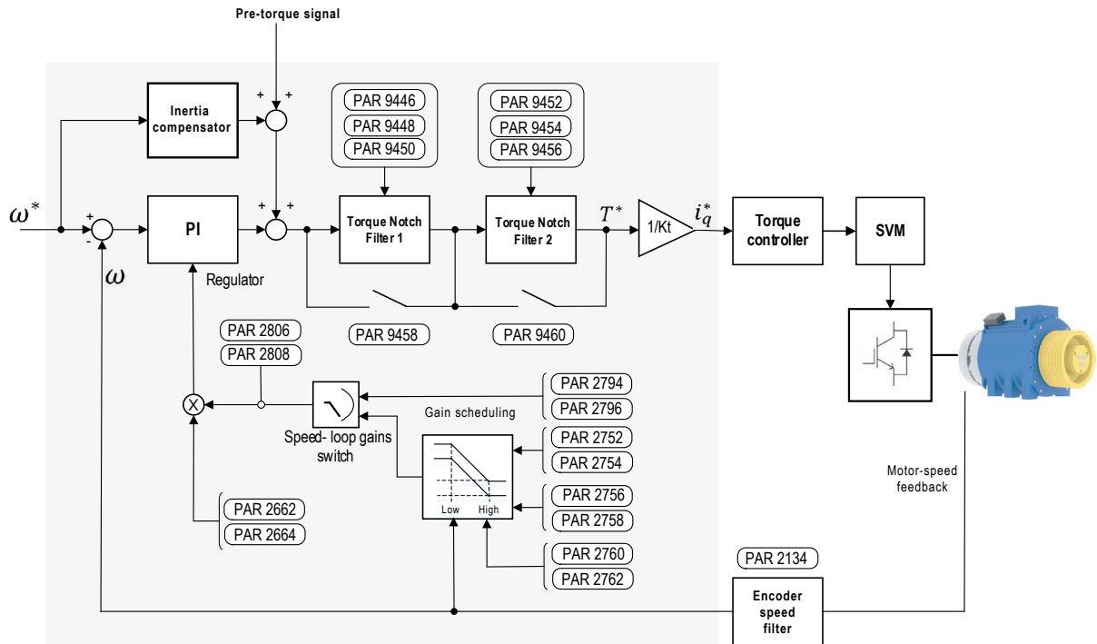
Figura 11.1: Schema a blocchi anello di controllo velocità motore
