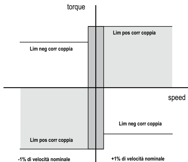
Limiti di coppia con Sel lim corr coppia = 2
