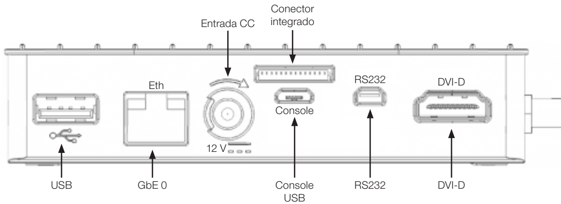
Figura 3.2: Superfície traseira
