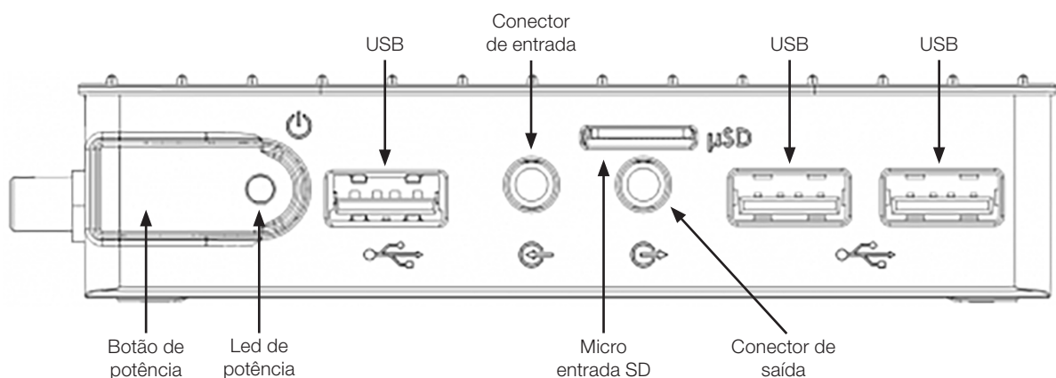
Figura 3.1: Superfície frontal
