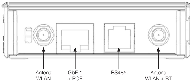
Figura 3.3: Superfície lateral
