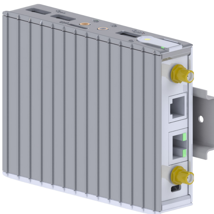
Figura 2.2: Fixação WCD-ED300 para trilho DIN (conjunto montado)
