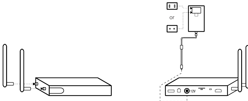
Figura 2.3: Conexão das antenas e do cabo de alimentação no WCD-ED300
