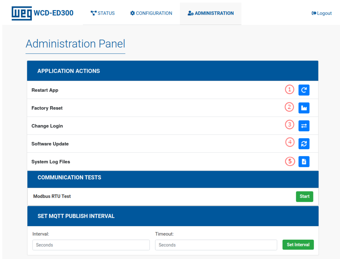
Figura 4.10: Página de administração - Ações de aplicação
