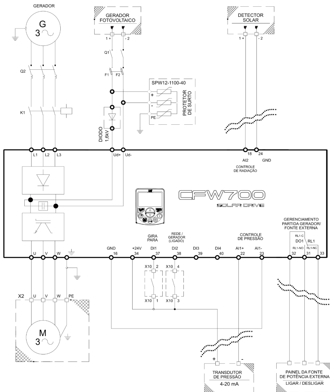
Figura 3.4– Esquema de ligação do sistema fotovoltaico de bombeamento de água para CFW700 modelo T4 com alimentação híbrida
