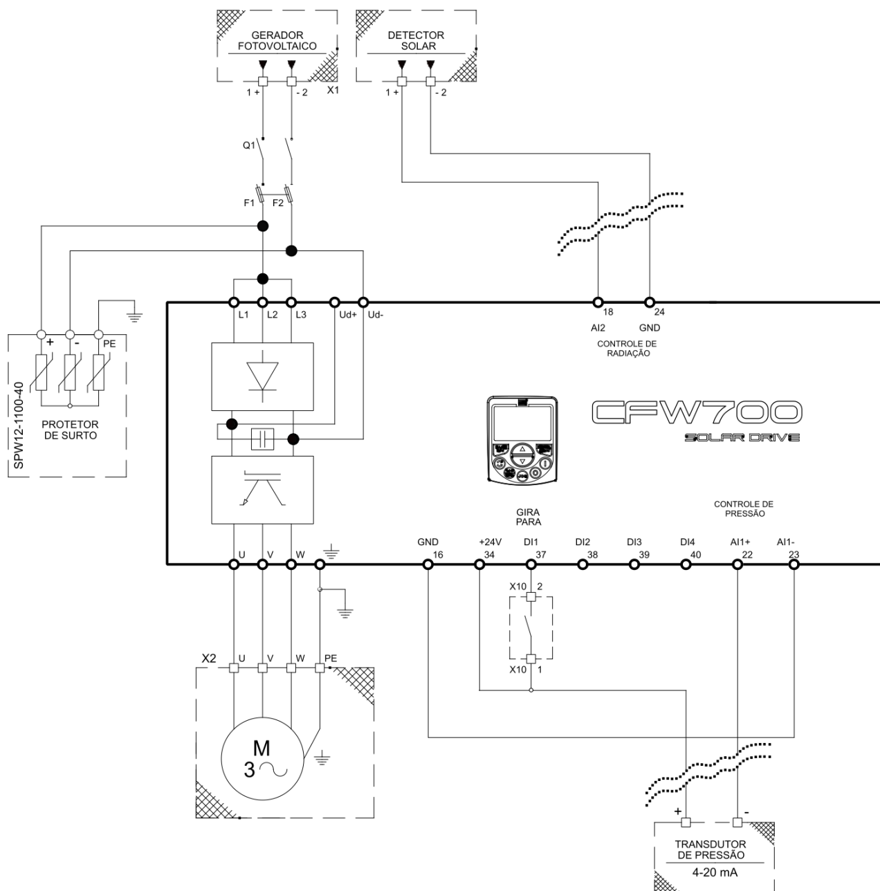
Figura 3.3 – Esquema de ligação do sistema fotovoltaico de bombeamento de água para CFW700 modelo T4
