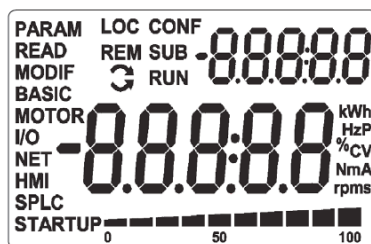
Figura 6.1 – Display da HMI ao energizar o drive
