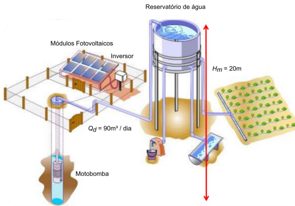
Figura 3.1 – Exemplo de sistema de bombeo fotovoltaico
