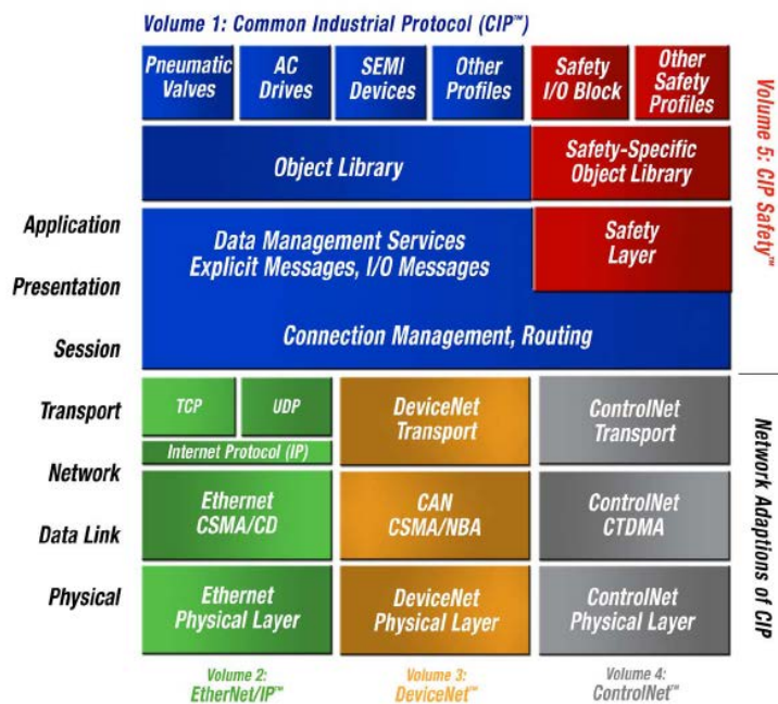
Figura 1.2: Estrutura em camadas do protocolo CIP
