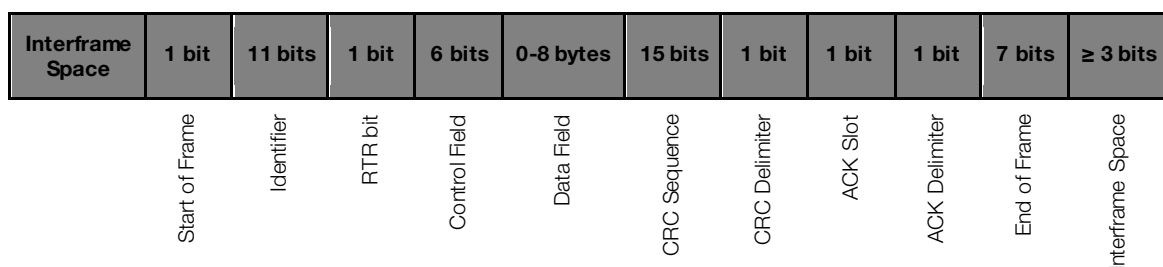
Figura 1.1: Frame de dados CAN
