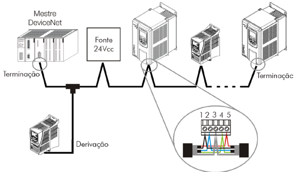
Figura 3.1: Exemplo de instalação em rede DeviceNet
