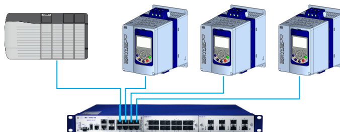
Figura 3.1: Topología en estrella
